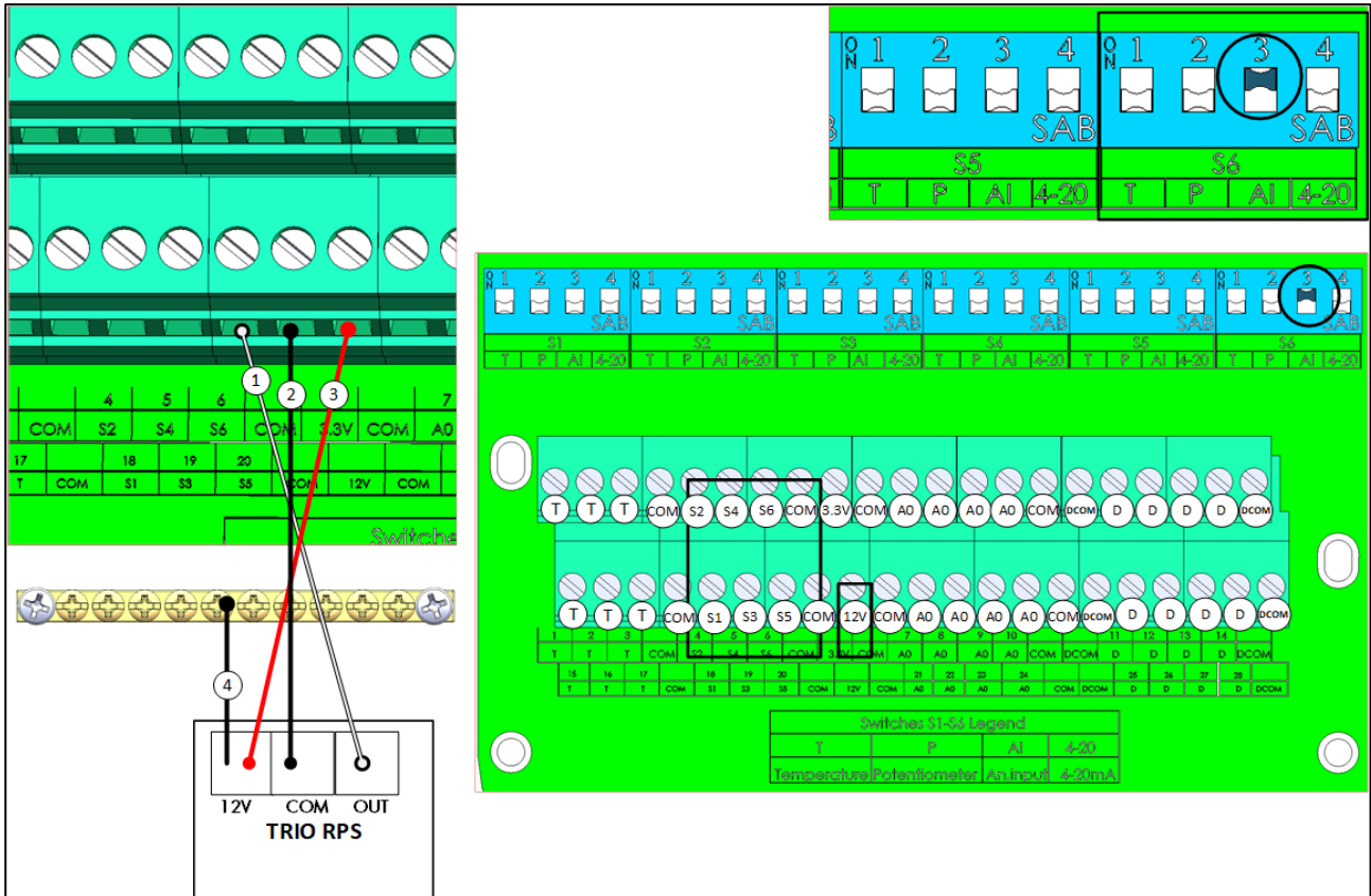
Figura 25: Fiação do RPS
