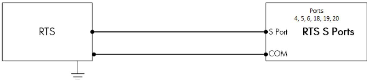
Figure 18: Diagrama esquemático da fiação do RTS Porta S
