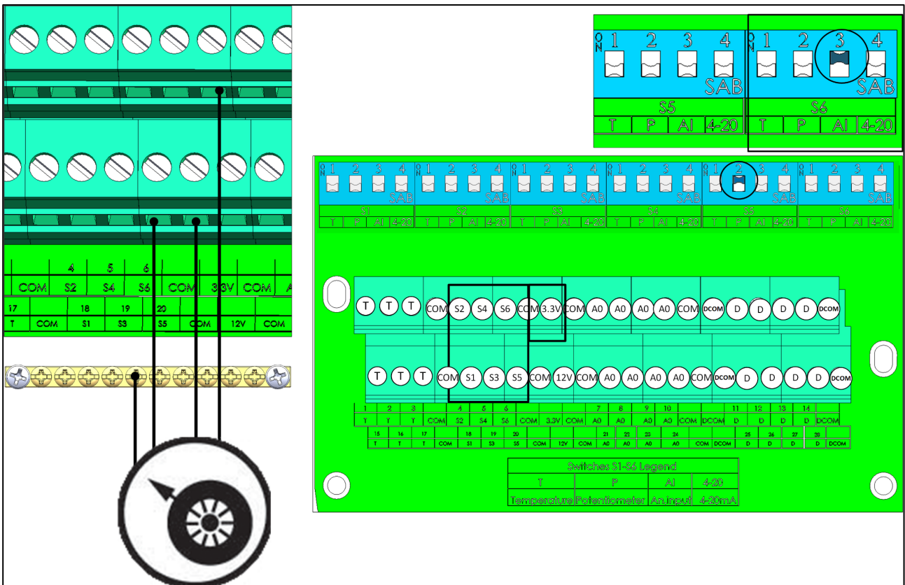
Figura 21: Fiação do potenciômetro
