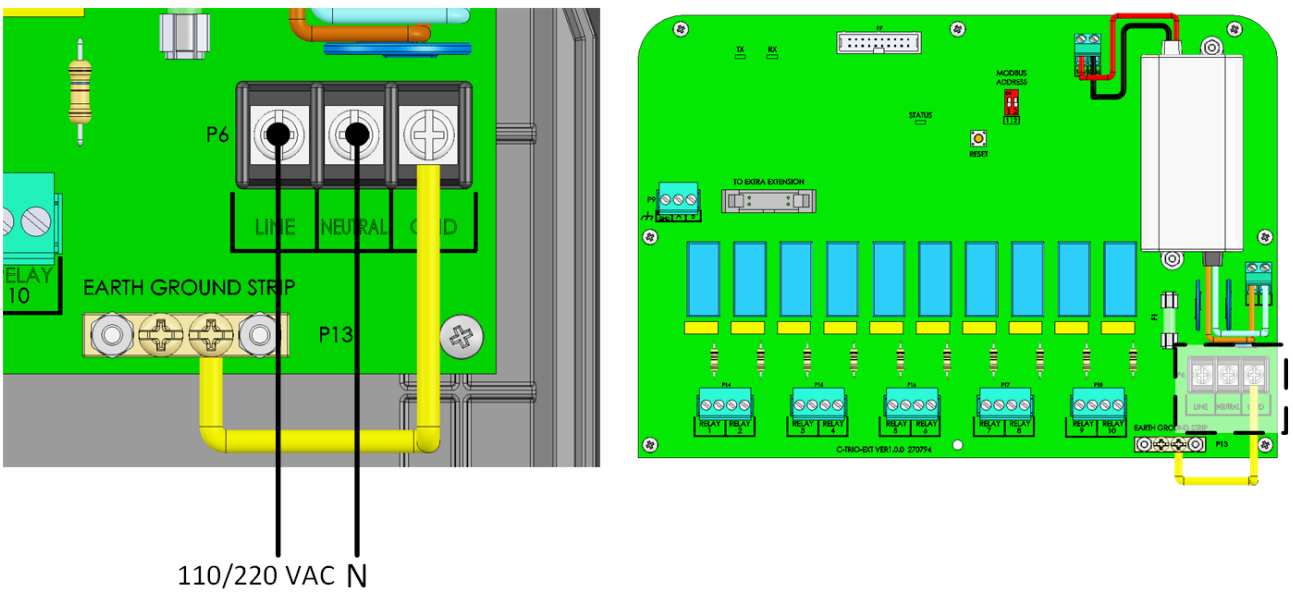
Figura 34: Portas de potência
