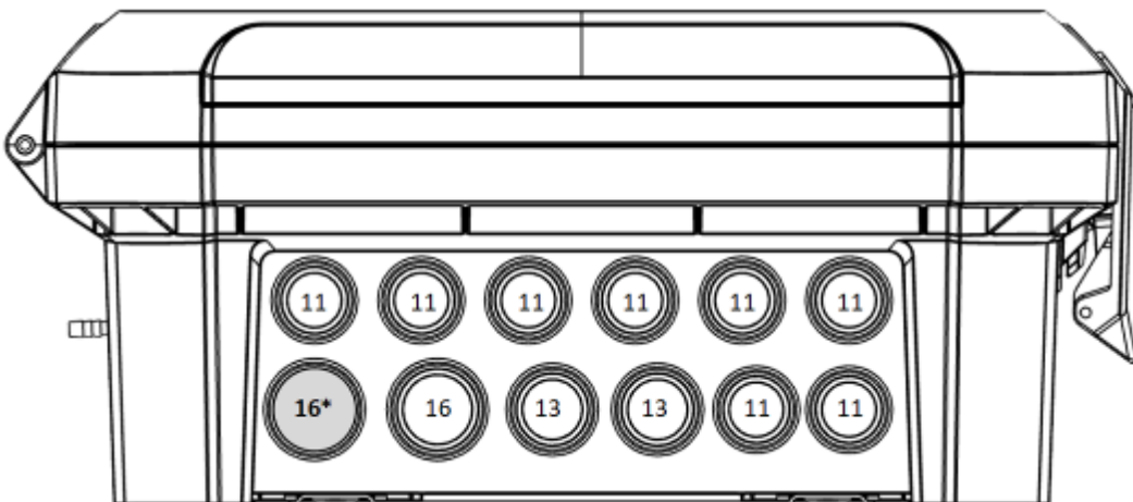
Figura 1: Separadores de cabos e tamanhos PG do Trio
