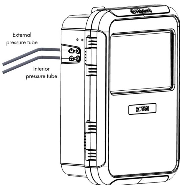
Figura 28: Mangueiras de pressão estáticas
