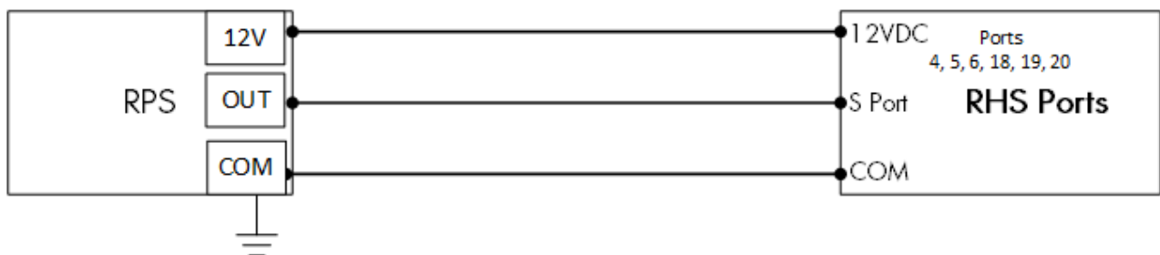
Figura 26: Diagrama esquemático da fiação do RPS
