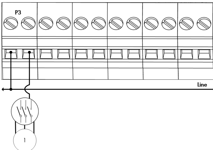
Figura 5: Visão detalhada da fiação dos relés
