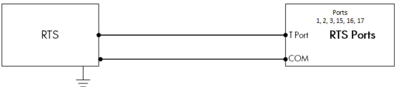
Figura 16: Diagrama esquemático da fiação do RTS
