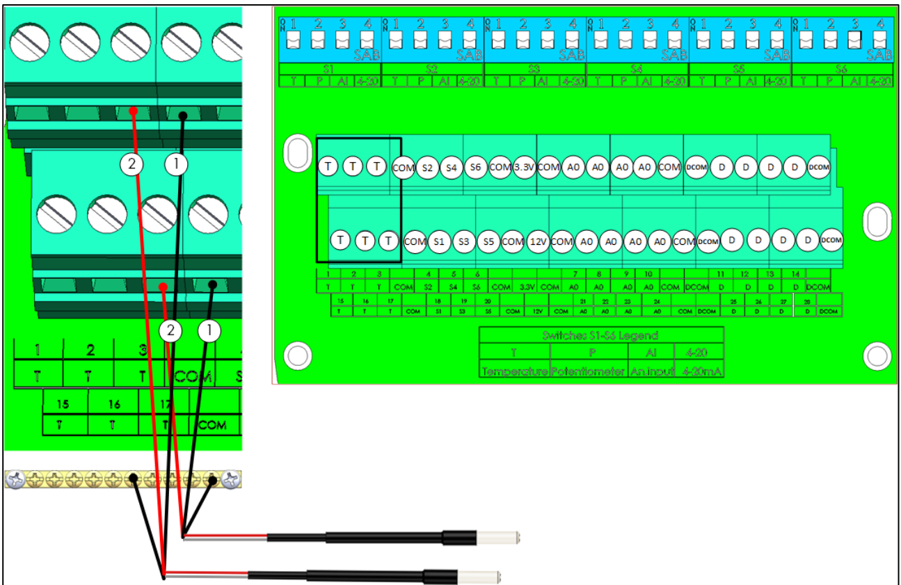
Figura 15: Fiação do RTS
