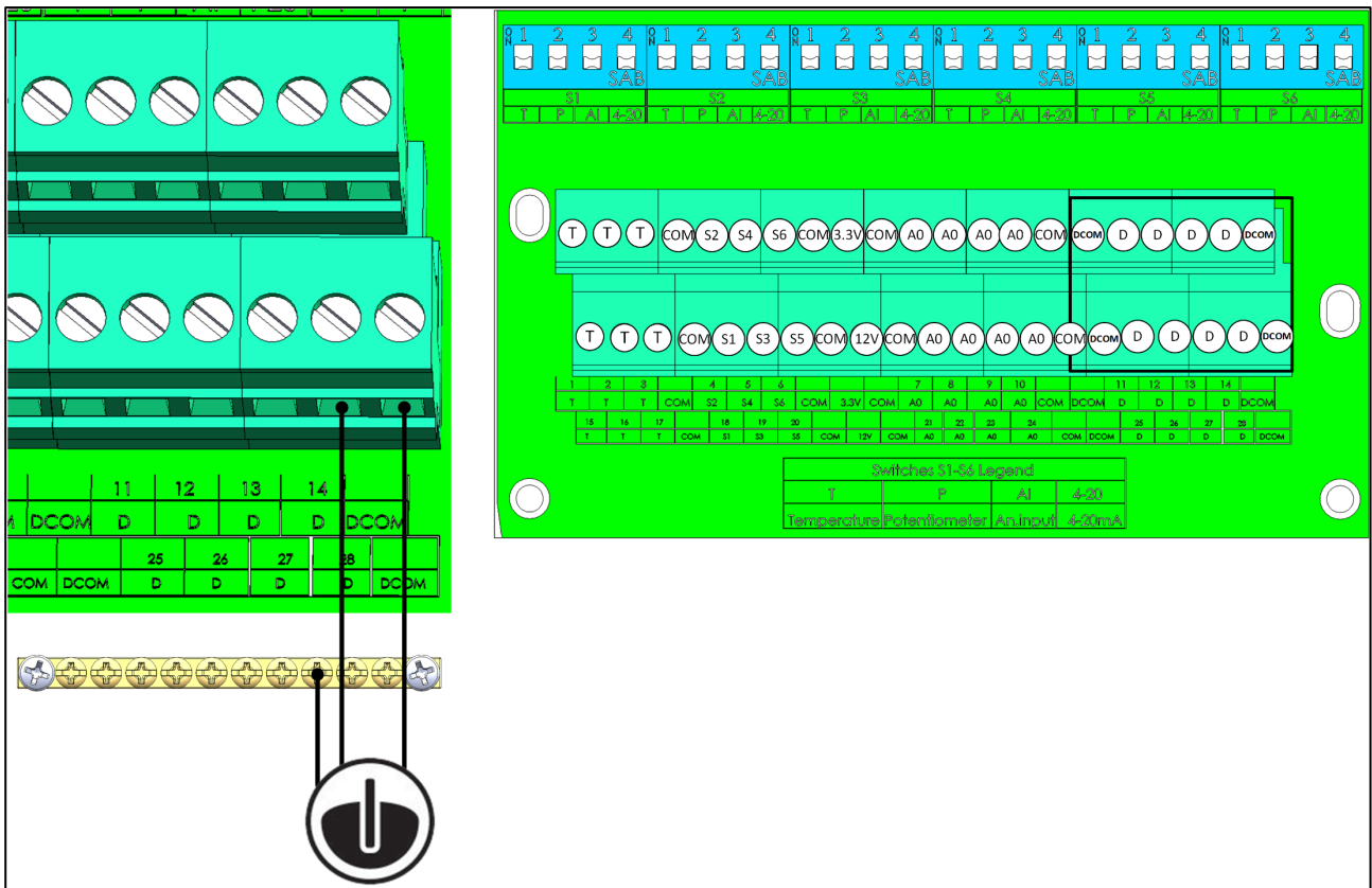
Figura 11: Dispositivos de entrada digitais (exemplo)
