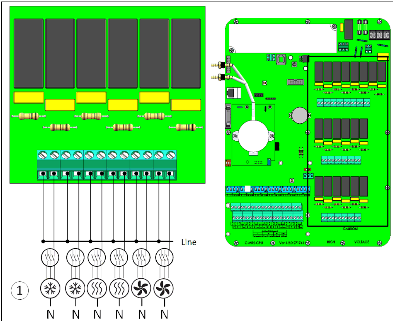
Figura 4: Dispositivos da alta tensão (exemplo)
