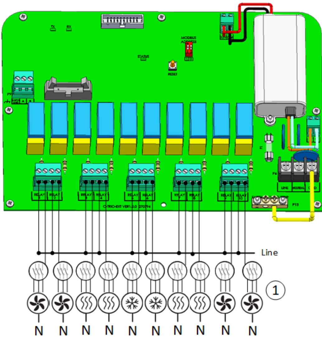
Figura 32: H Dispositivos da alta tensão (exemplos)
