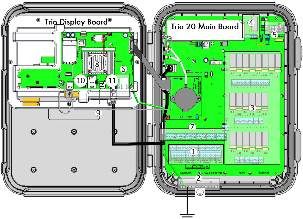
Figura 2: Layout do quadro
