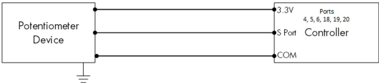
Figura 22: Diagrama esquemático da fiação do potenciômetro
