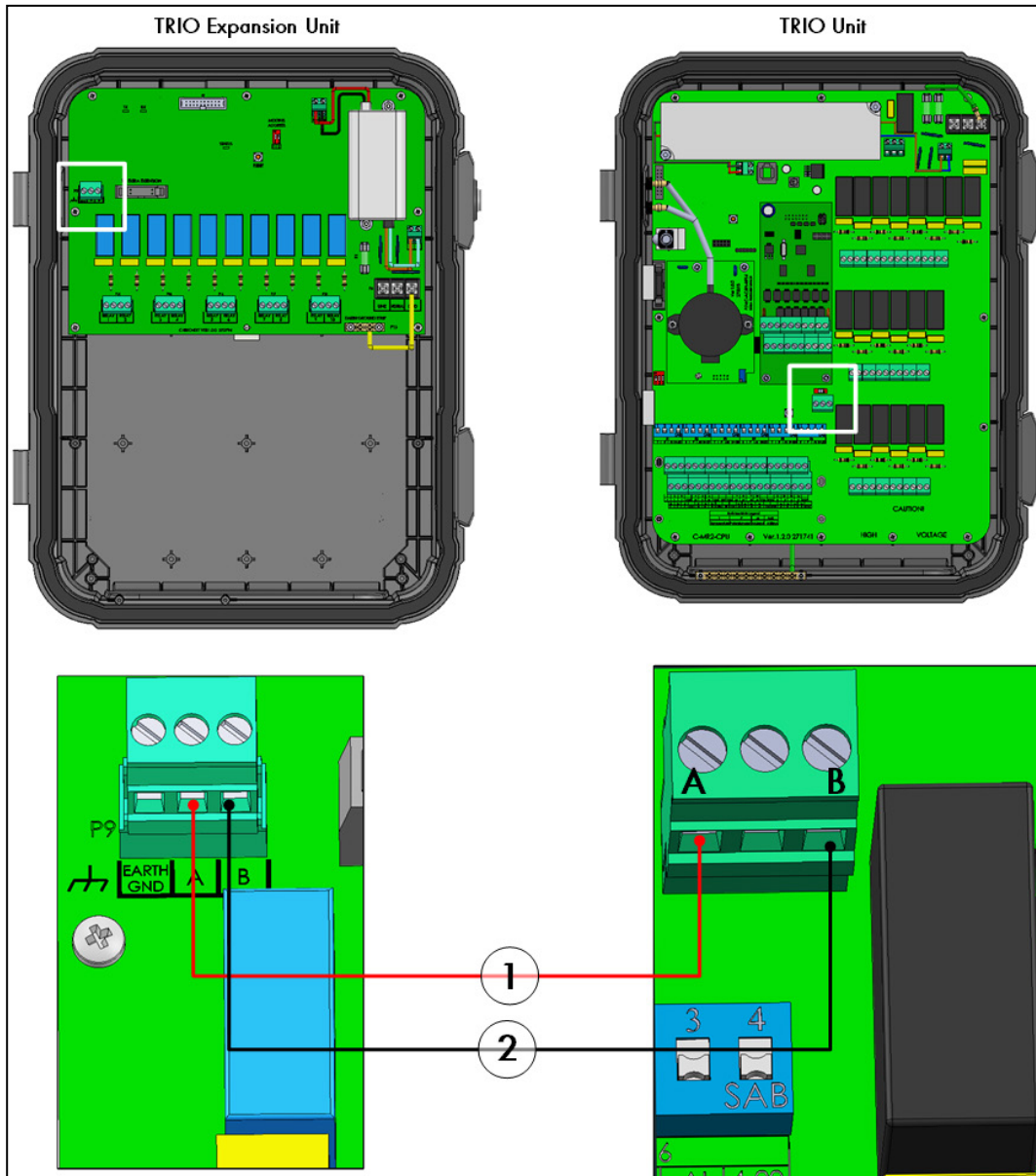
Figura 31: Diagrama de fiação
