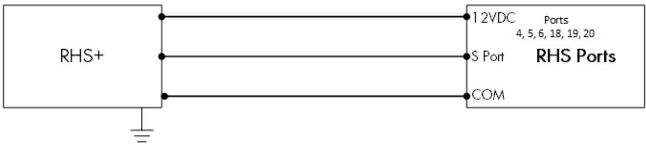
Figura 20: Diagrama esquemático da fiação sensor RHS+
