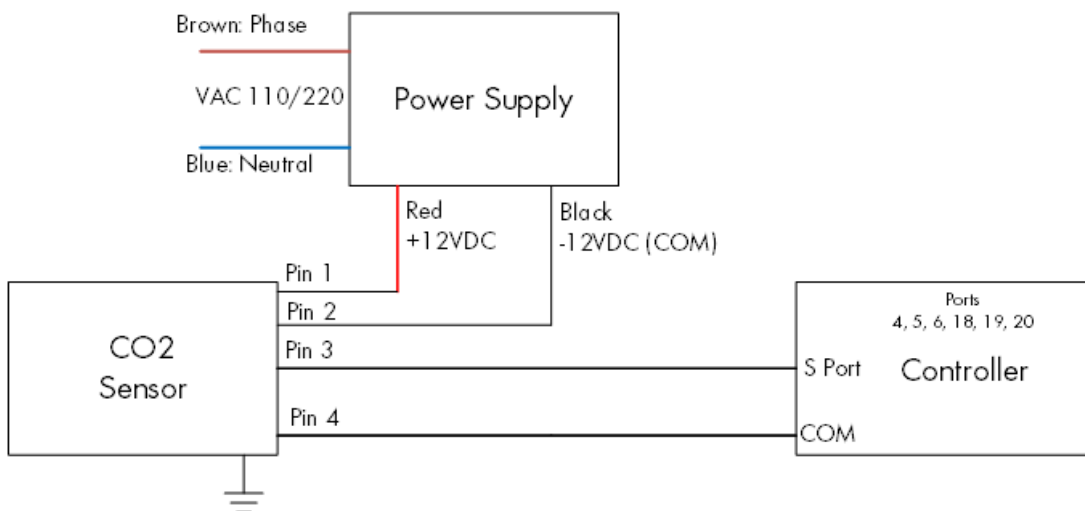
Figura 14: Diagrama esquemático da fiação do sensor de CO 2
