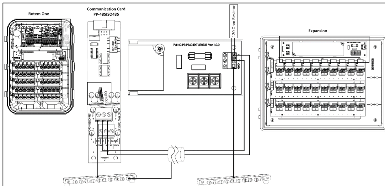
Figura 4: Fiação da expansão Platinum Pro para Platinum Expansion
