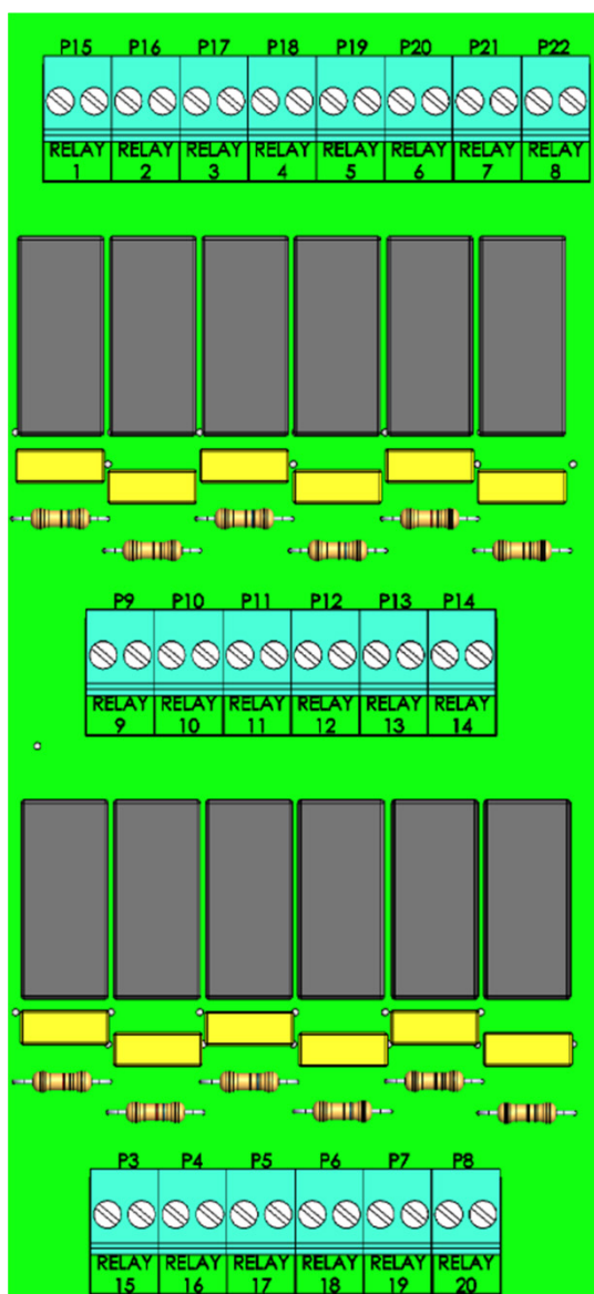
Figura 7: Numerazione di relè (relay) e porte
