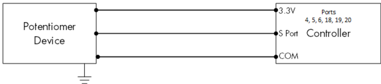
Figura 23: Schema di cablaggio del potenziometro (potentiometer device)
