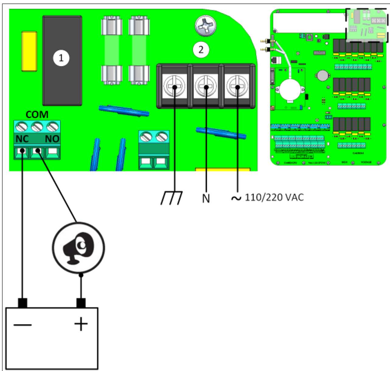
Figura 8: Relè di allarme e Porte di alimentazione
