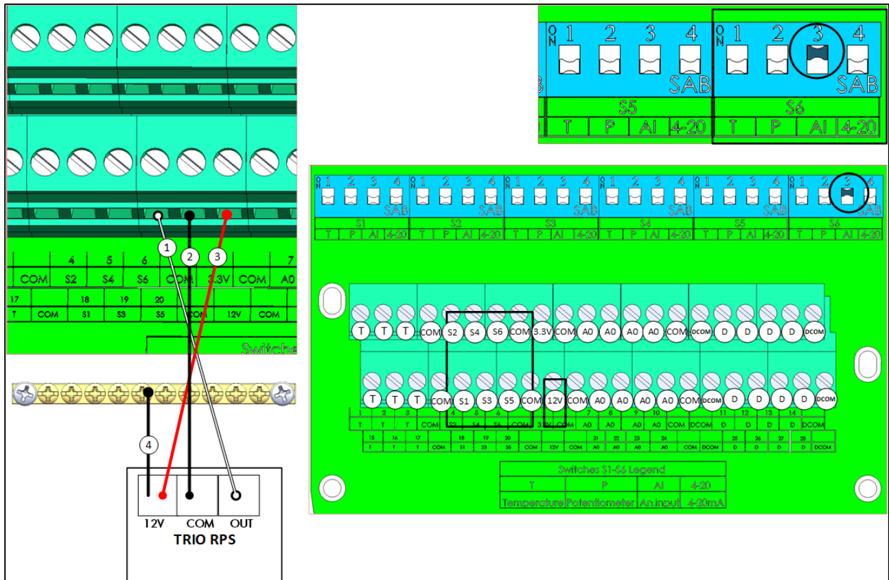
Figura 26: Cablaggio RPS
