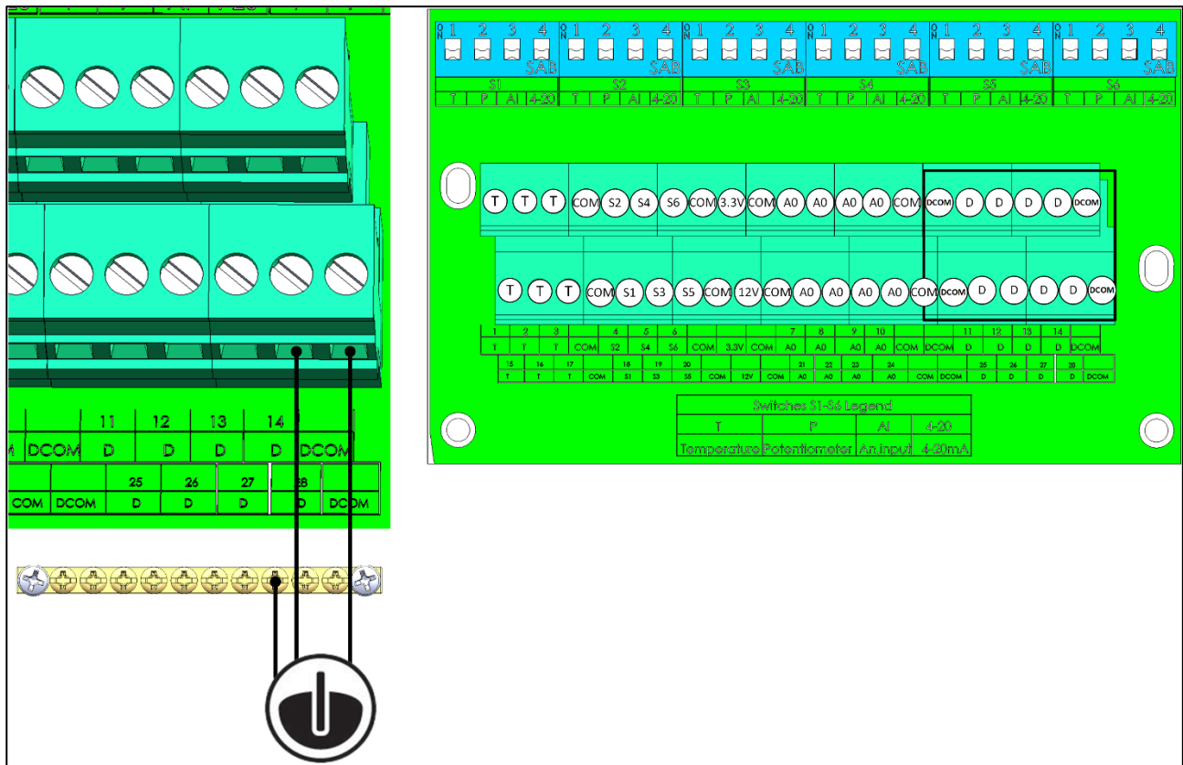
Figura 12: dispositivi di ingresso digitale (esempi)
