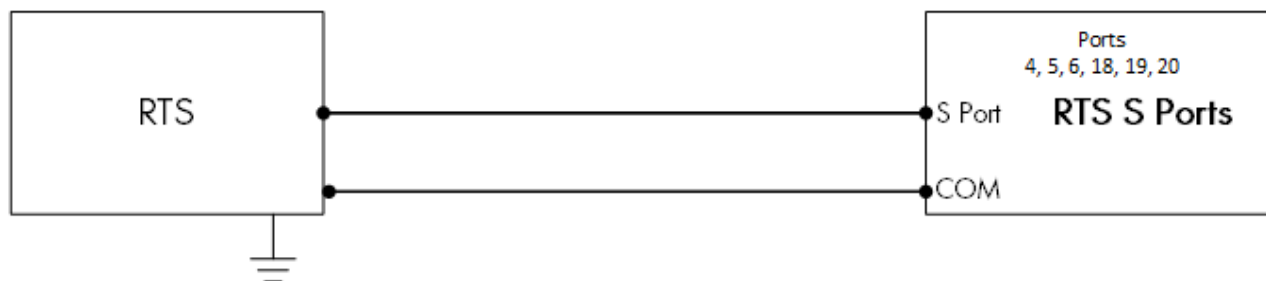
Figura 19: Schema di cablaggio RTS S-Porta
