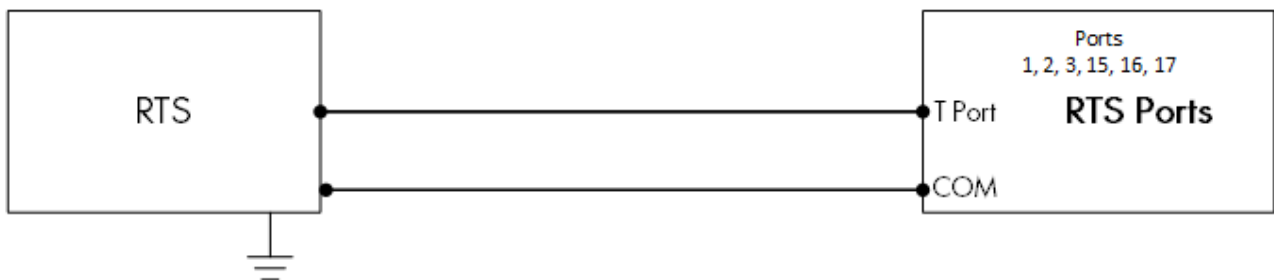
Figura 17: Schema di cablaggio RTS
