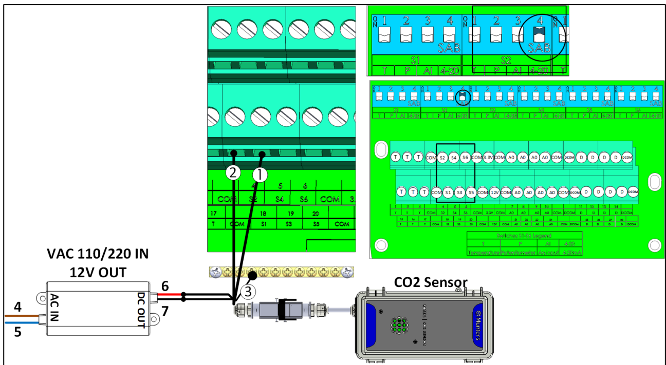
Figura 14: Cablaggio del Sensore di CO2
