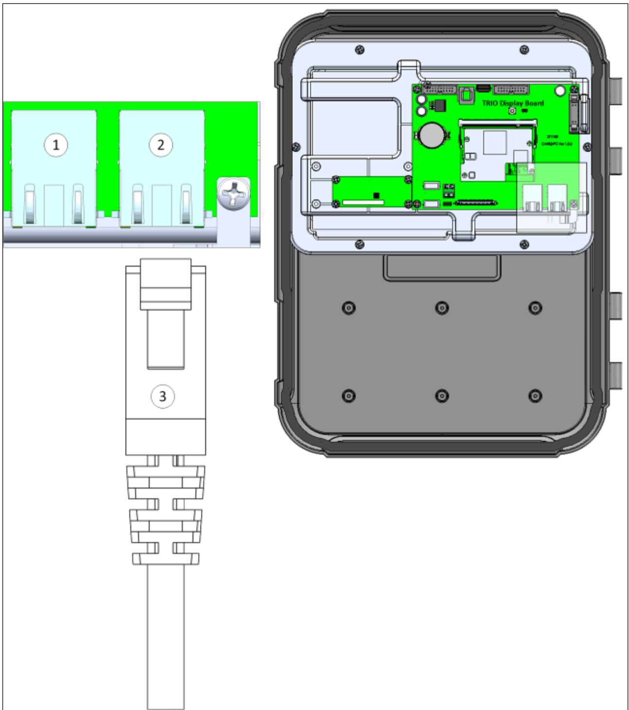
Figura 9: Porta Ethernet
