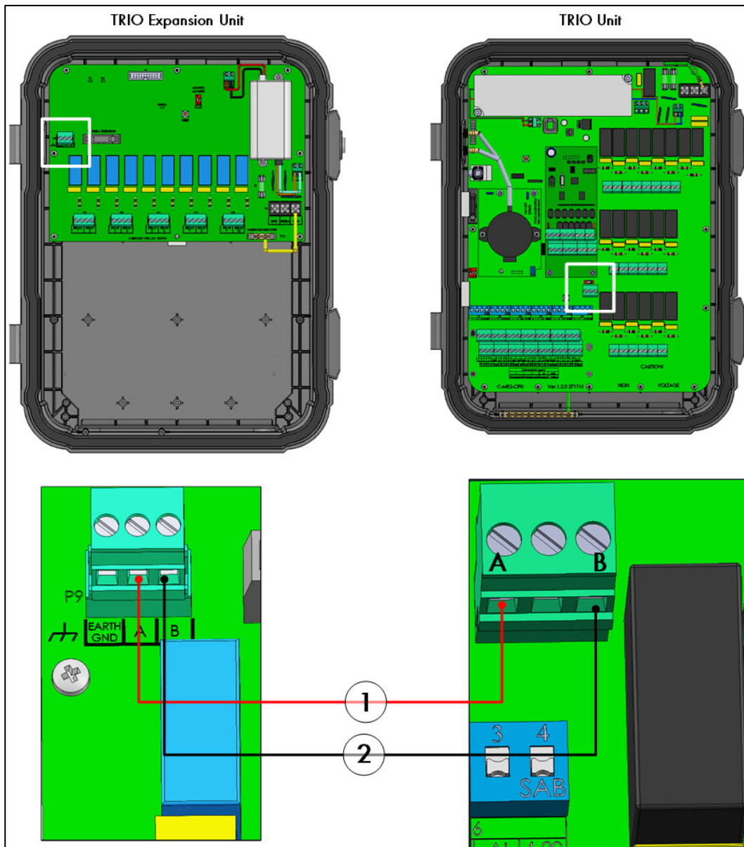
Figura 32: Schema elettrico
