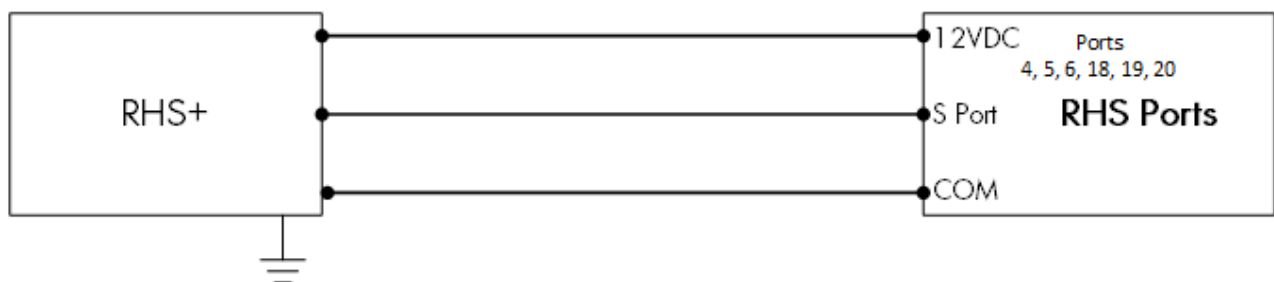
Figura 21: Schema di cablaggio del sensore RHS+
