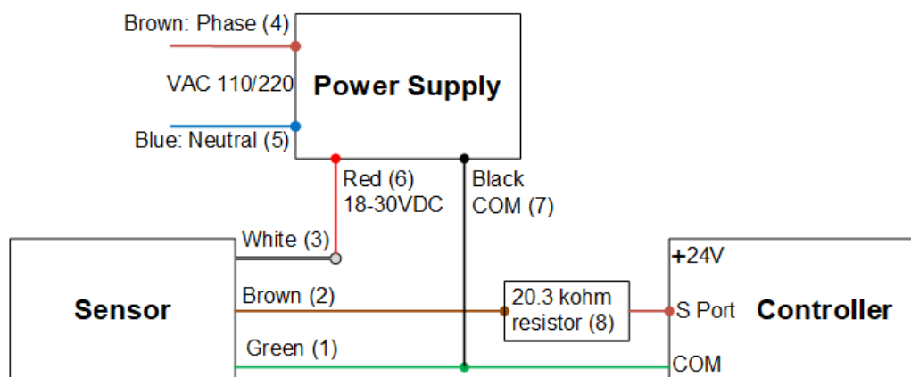
Figura 25: Schema di Cablaggio del Sensore (Sensor) Ammoniaca
