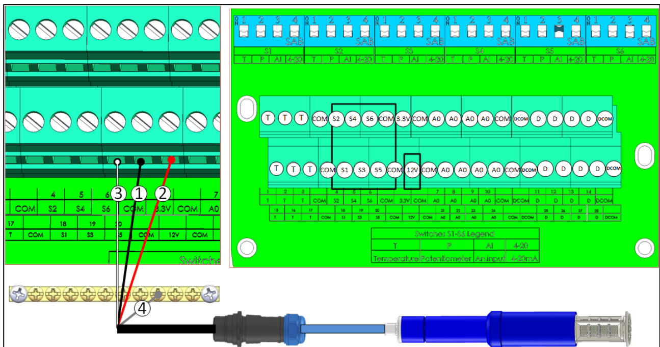
Figura 20: Cablaggio RHS+
