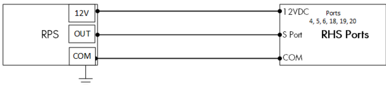
Figura 27: Schema del cablaggio RPS
