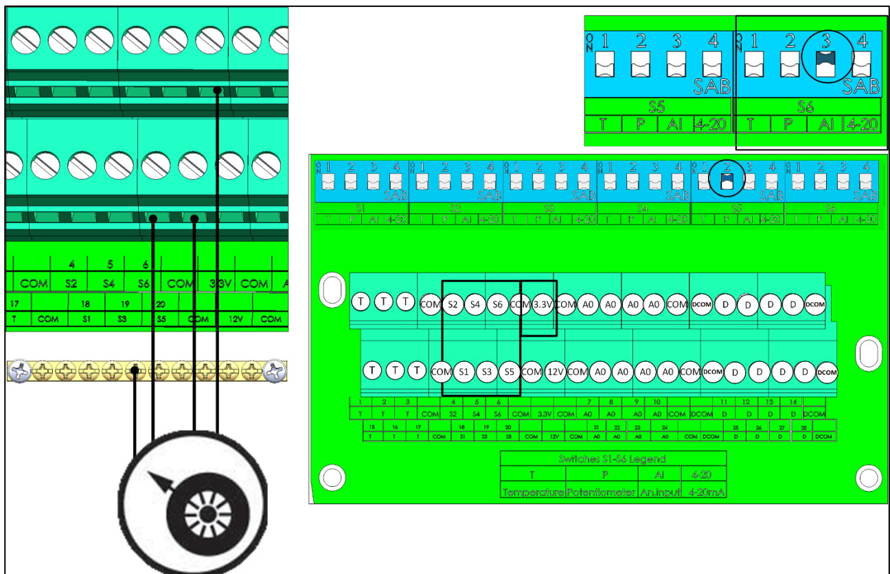
Figura 22: Cablaggio potenziometro
