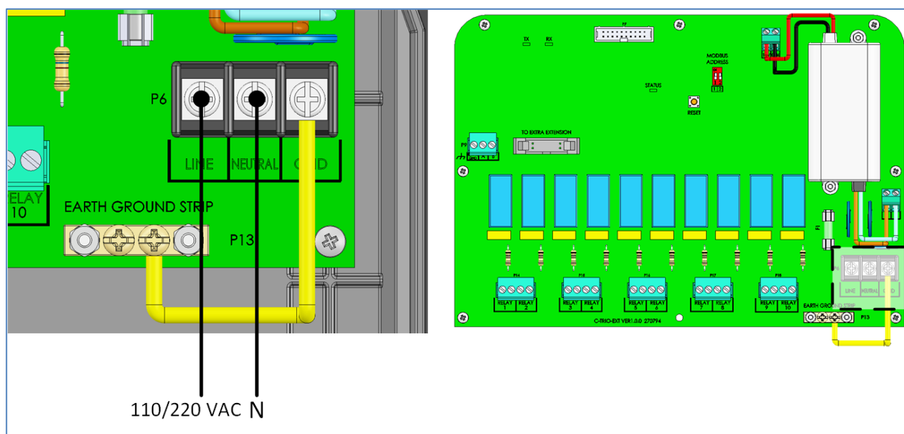
Figura 35: Porte di alimentazione
