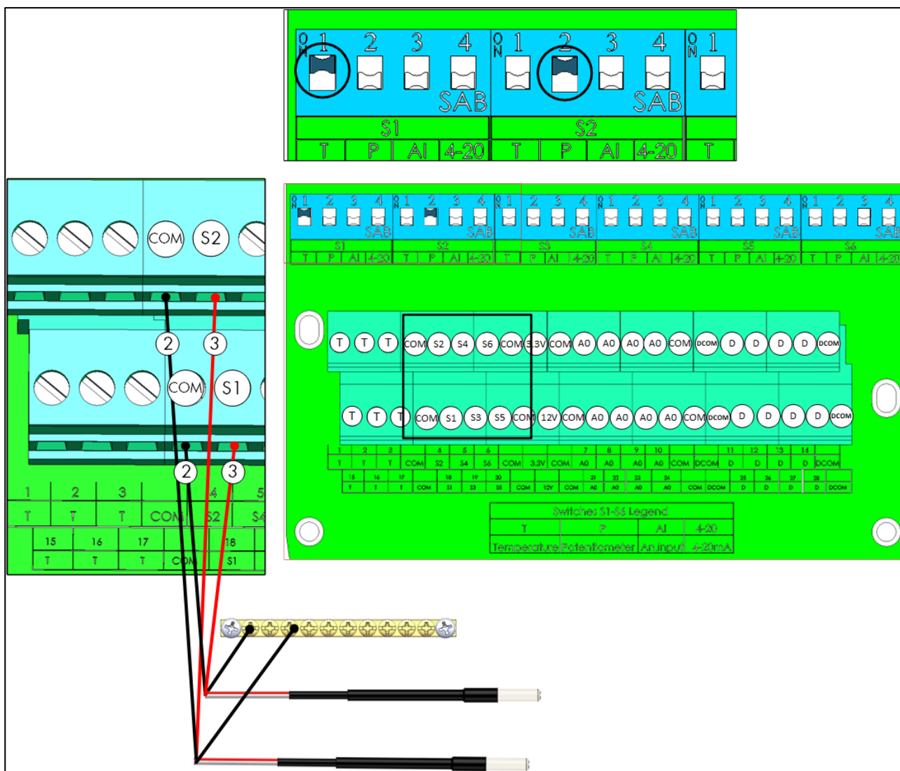
Figura 18: Schema di cablaggio RTS S-Porta
