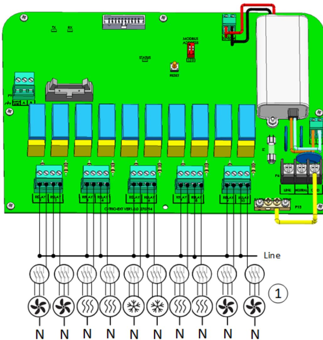
Figura 33: Dispositivi ad alta tensione (esempi)
