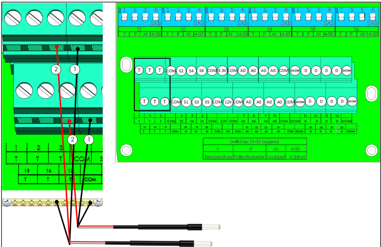
Figura 16: Cablaggio RTS
