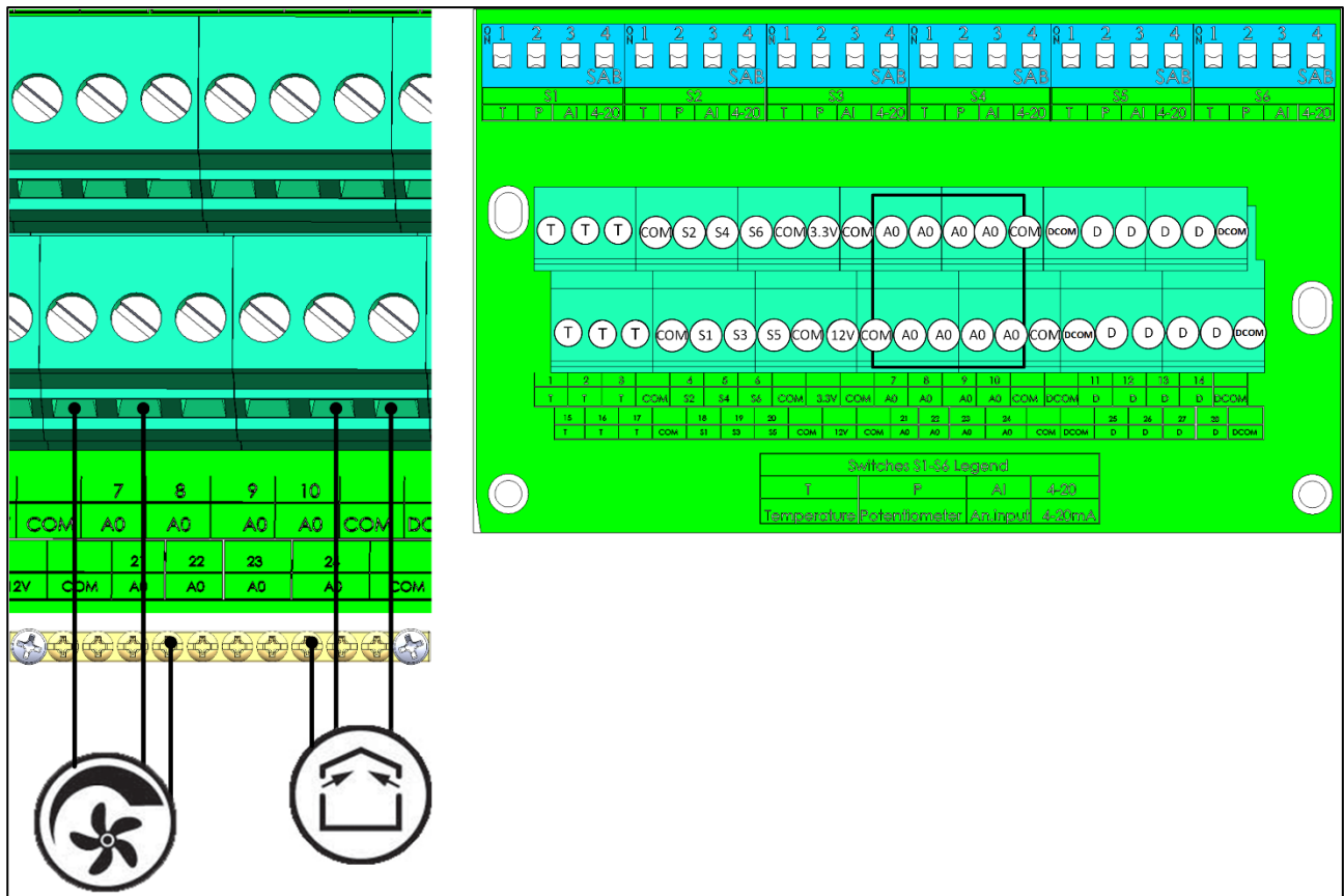
Figura 10: Dispositivi di uscita analogica (esempi)
