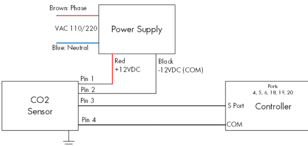
Figura 15: Schema di cablaggio del sensore di CO2
