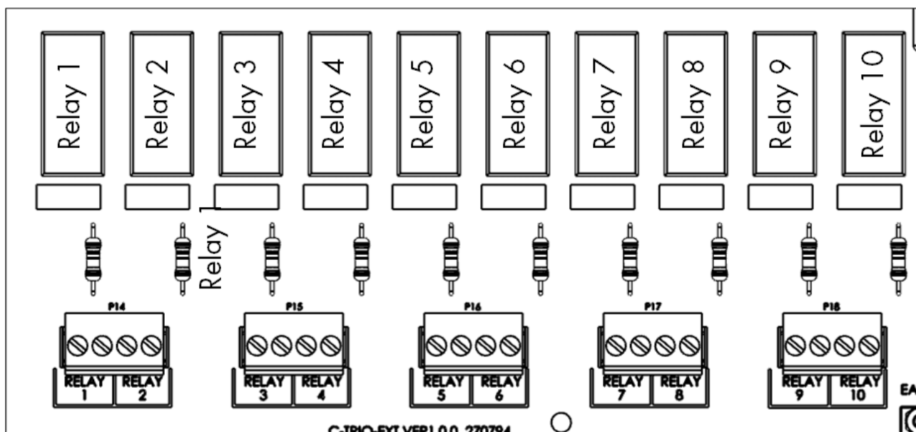
Figura 34: Numerazione di relè (relay) e porte
