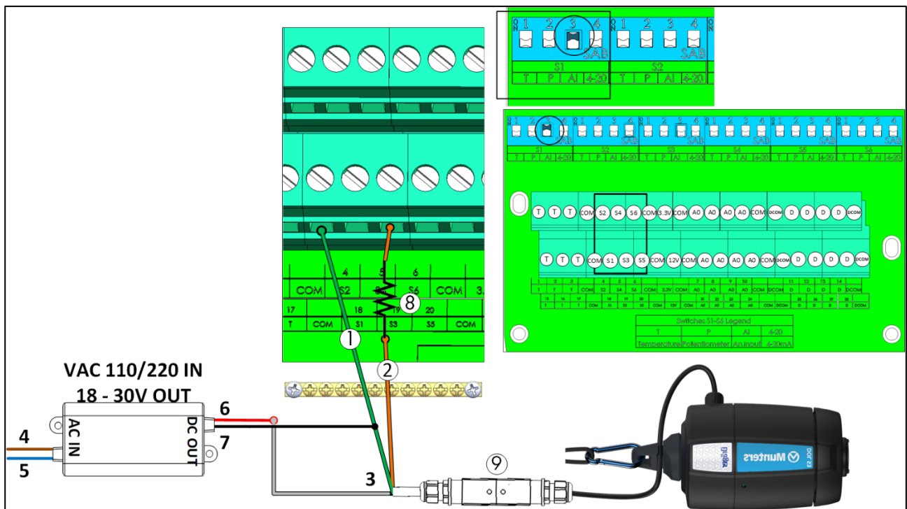
Figura 24: Cablaggio del Sensore di Ammoniaca
