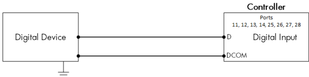
Figura 13: Schema di cablaggio del dispositivo digitale (digital)
