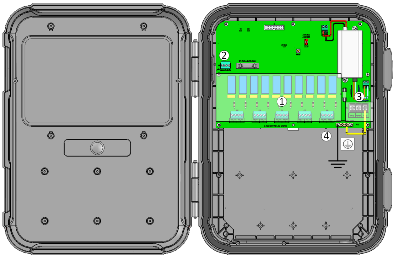
Figura 31: Layout della scheda
