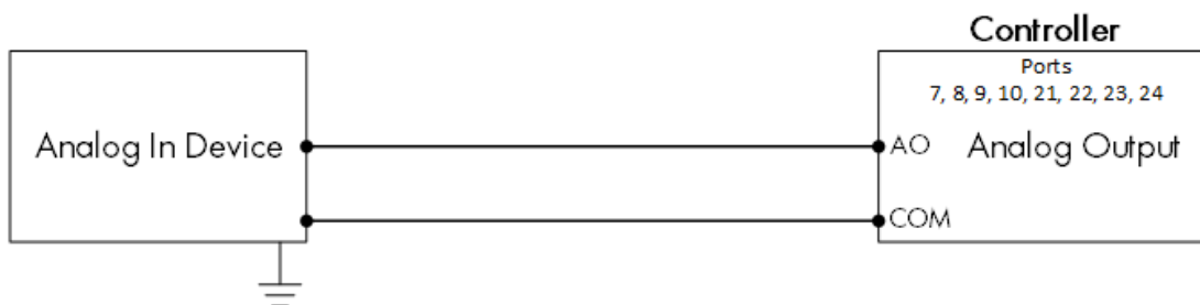
Figura 11: Schema di cablaggio del dispositivo analogico (analog)
