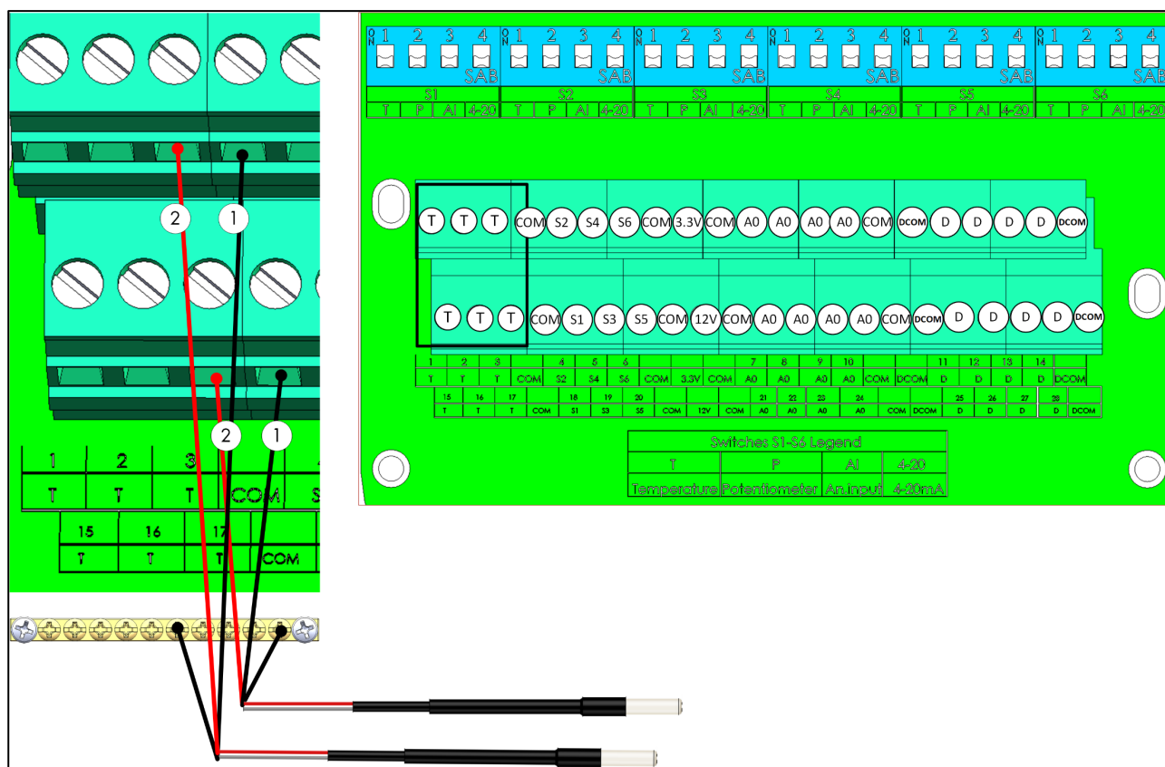
Figur 23: Ledningsføring for RTS-2
