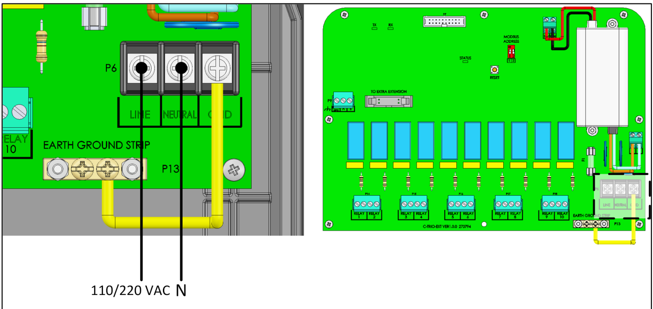
Figur 64: Strømporte
