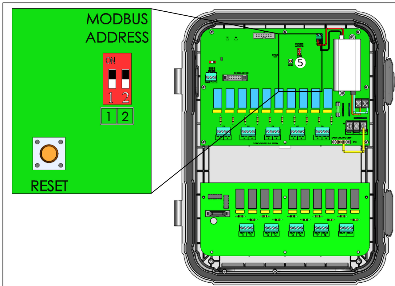
Figur 61: Ekspansionsadresse
