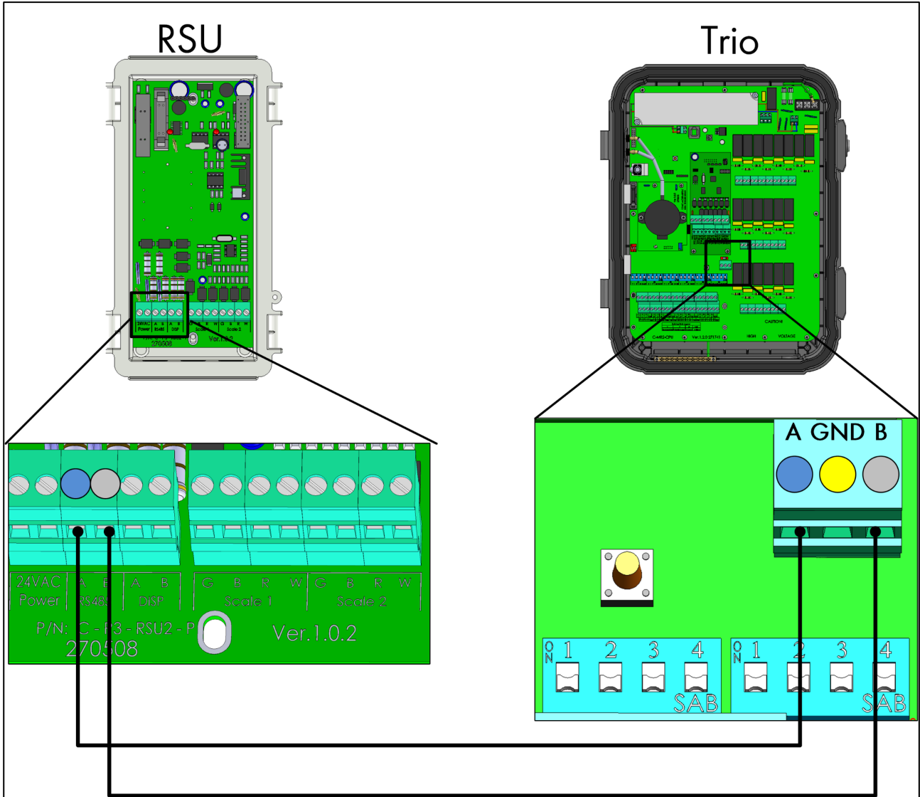
Figur 43: Trio – RSU-ledningsføring
