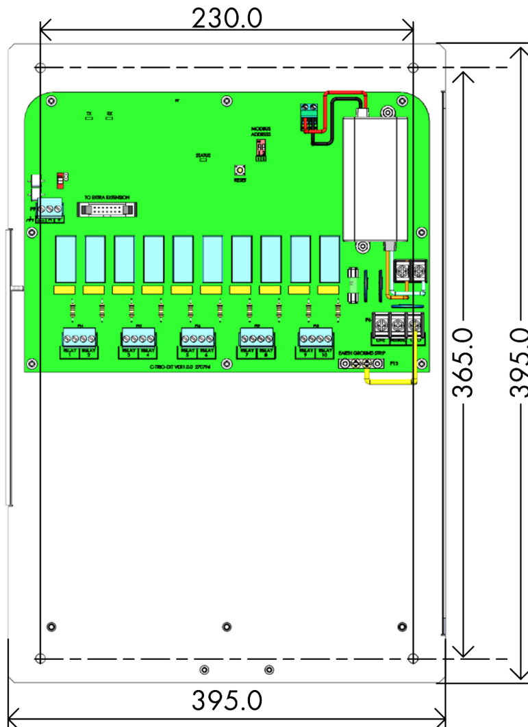
Figur 80: Expansion – bagpaneldimensioner
