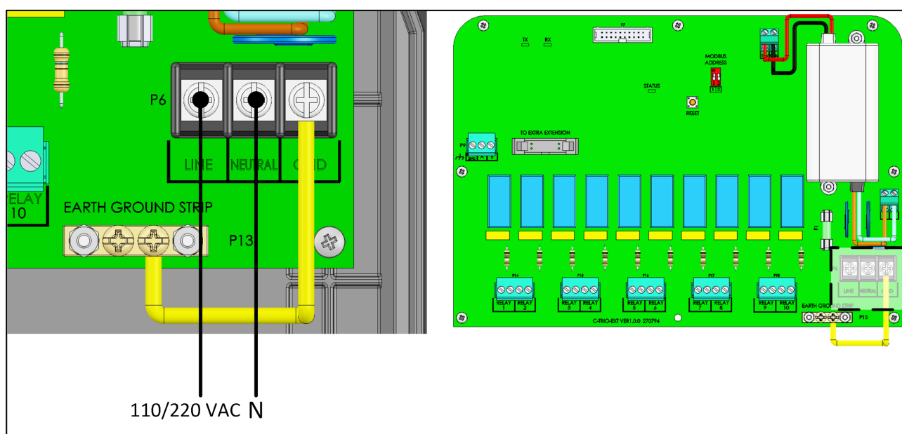
Figur 58: Strømporte
