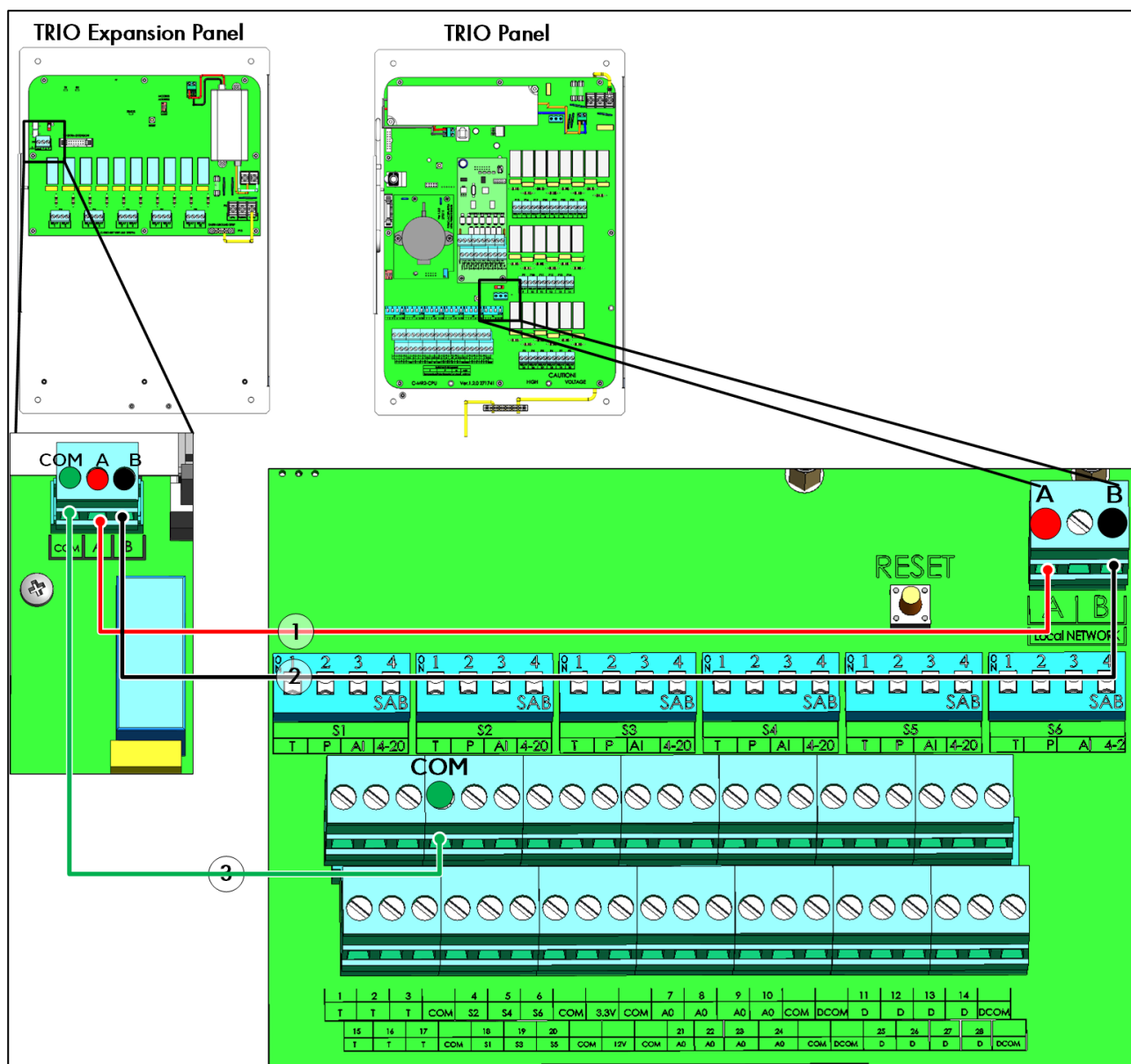
Figur 82: Kabelføring for panelmontering/ekspansionspanelmontering
