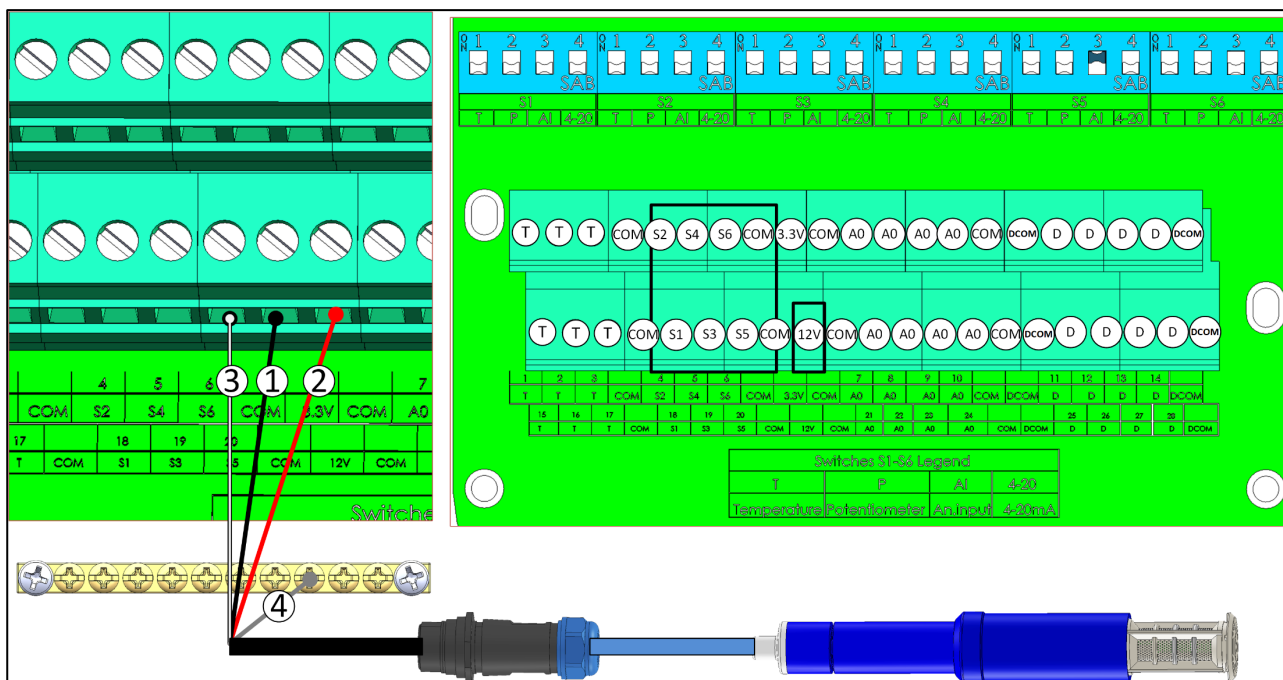
Figur 27: RHS+ -ledninger
