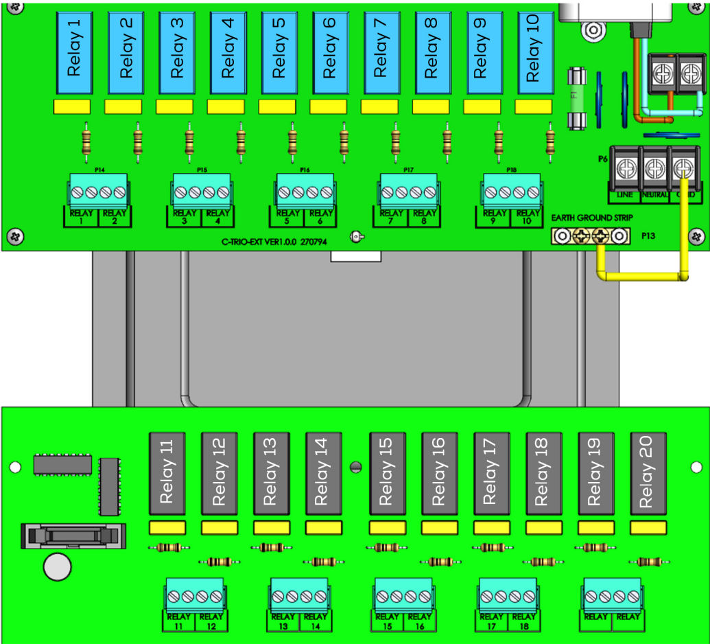
Figur 63: Relæ- og portnummerering
