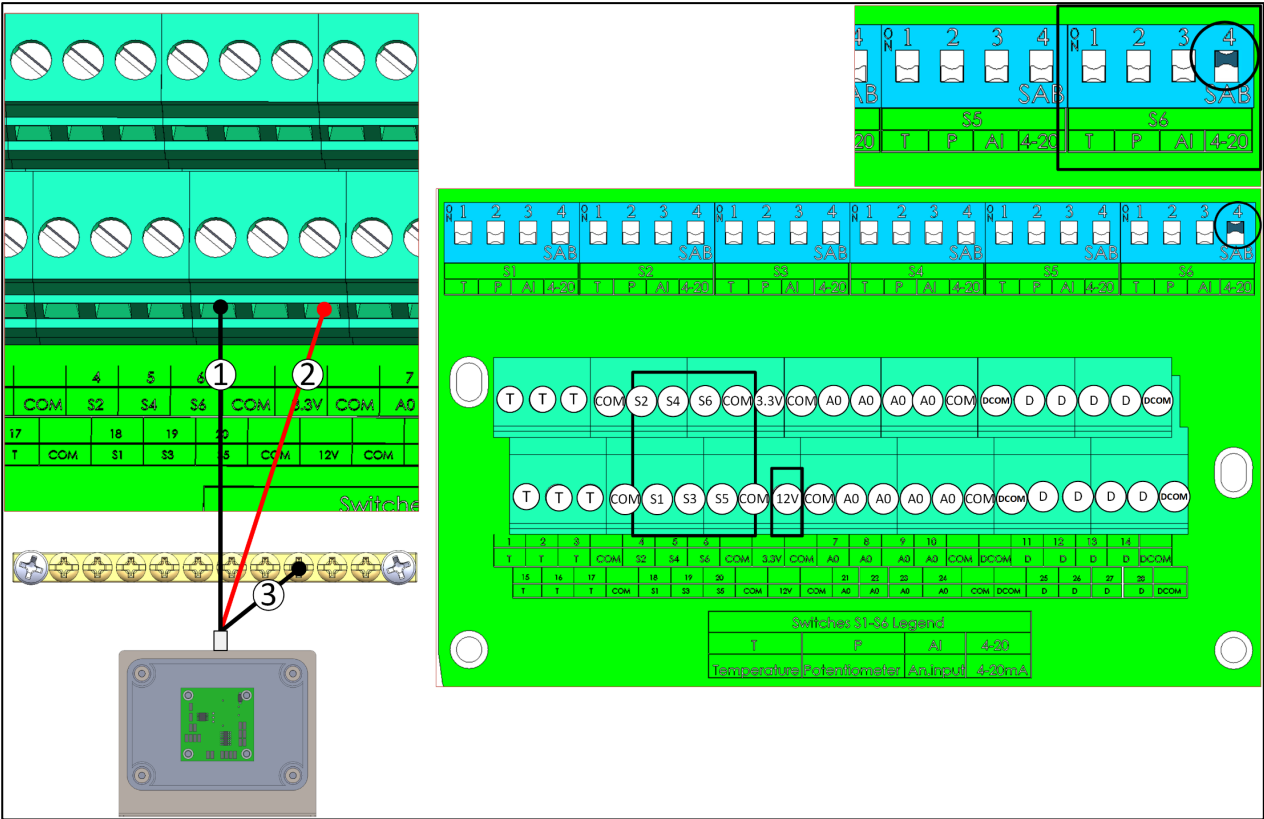
Figur 34: Lyssensor-ledninger
