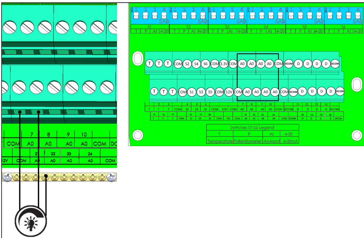
Figur 16: Lysdæmperenheder
