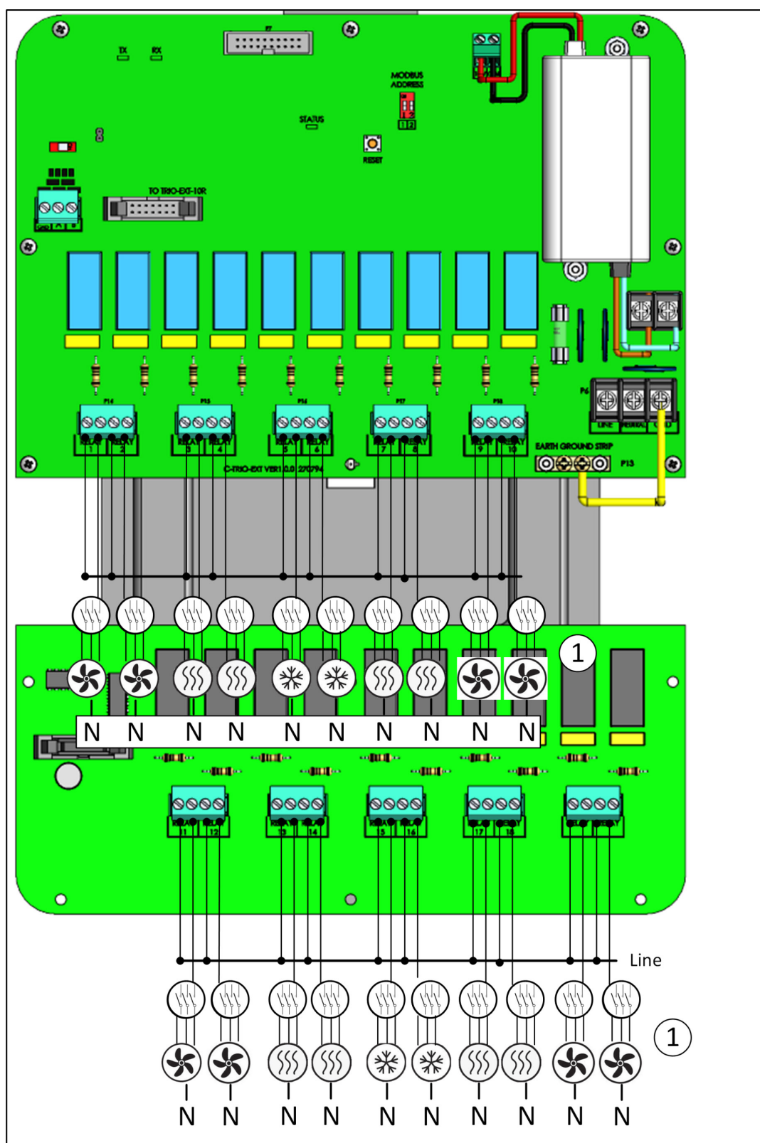
Figur 62: Højspændingsenheder (eksempler)
