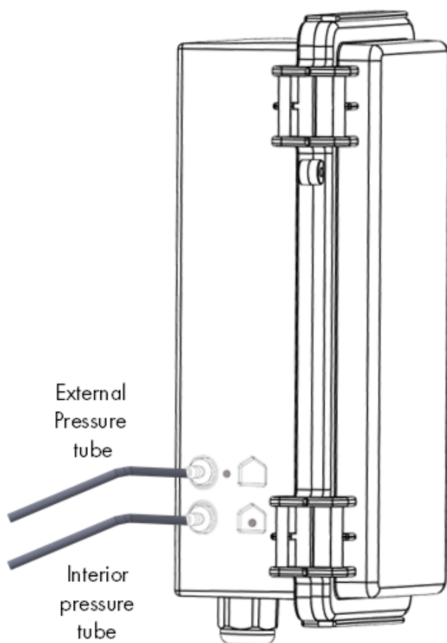
Figur 38: Slange til statisk tryk
