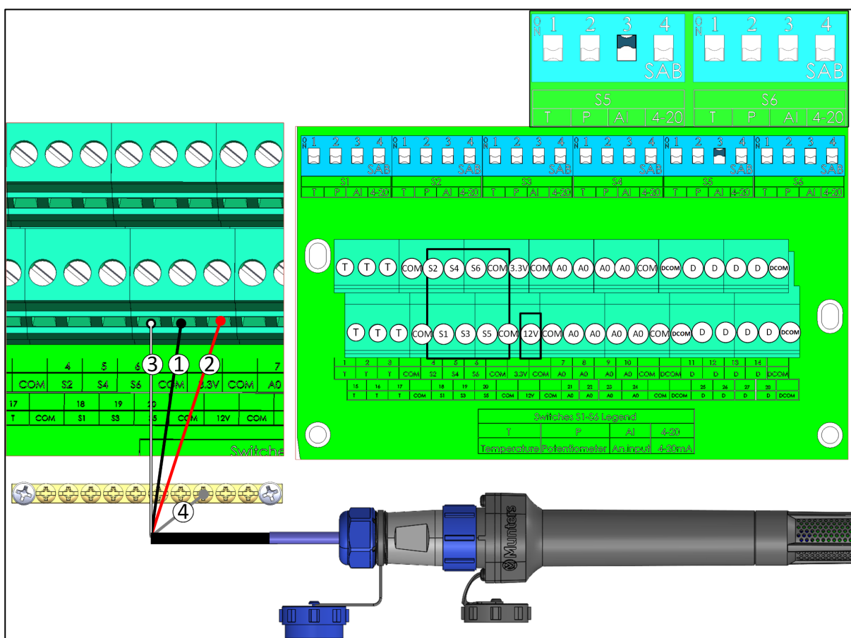
Figur 28: RHS -ledninger
