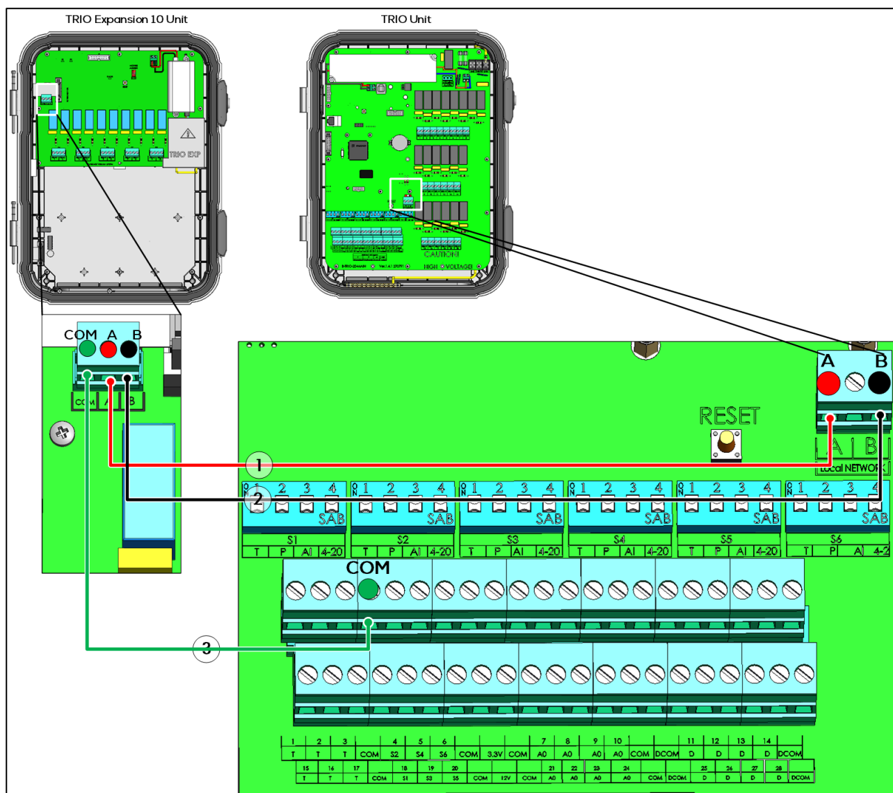
Figur 54: Ledningsdiagram
