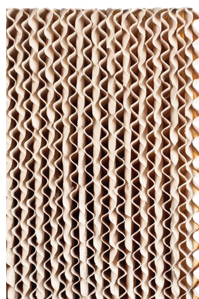
GLASdek GX30
