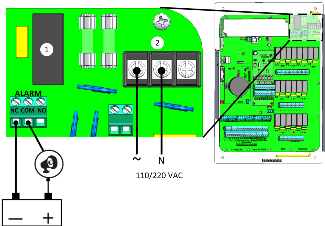
图 49: 报警继电器和电源端口
