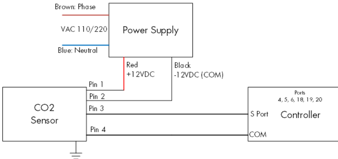
图 15:二氧化碳传感器接线图
