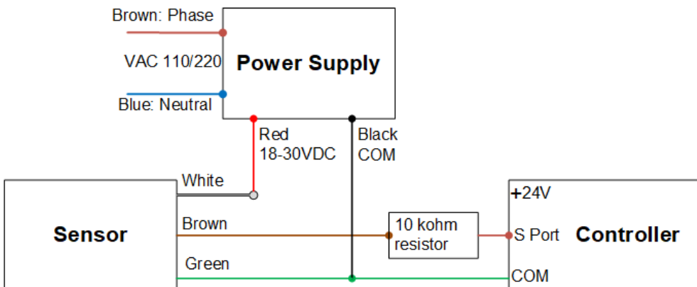
图 24: 氨气传感器接线示意图
