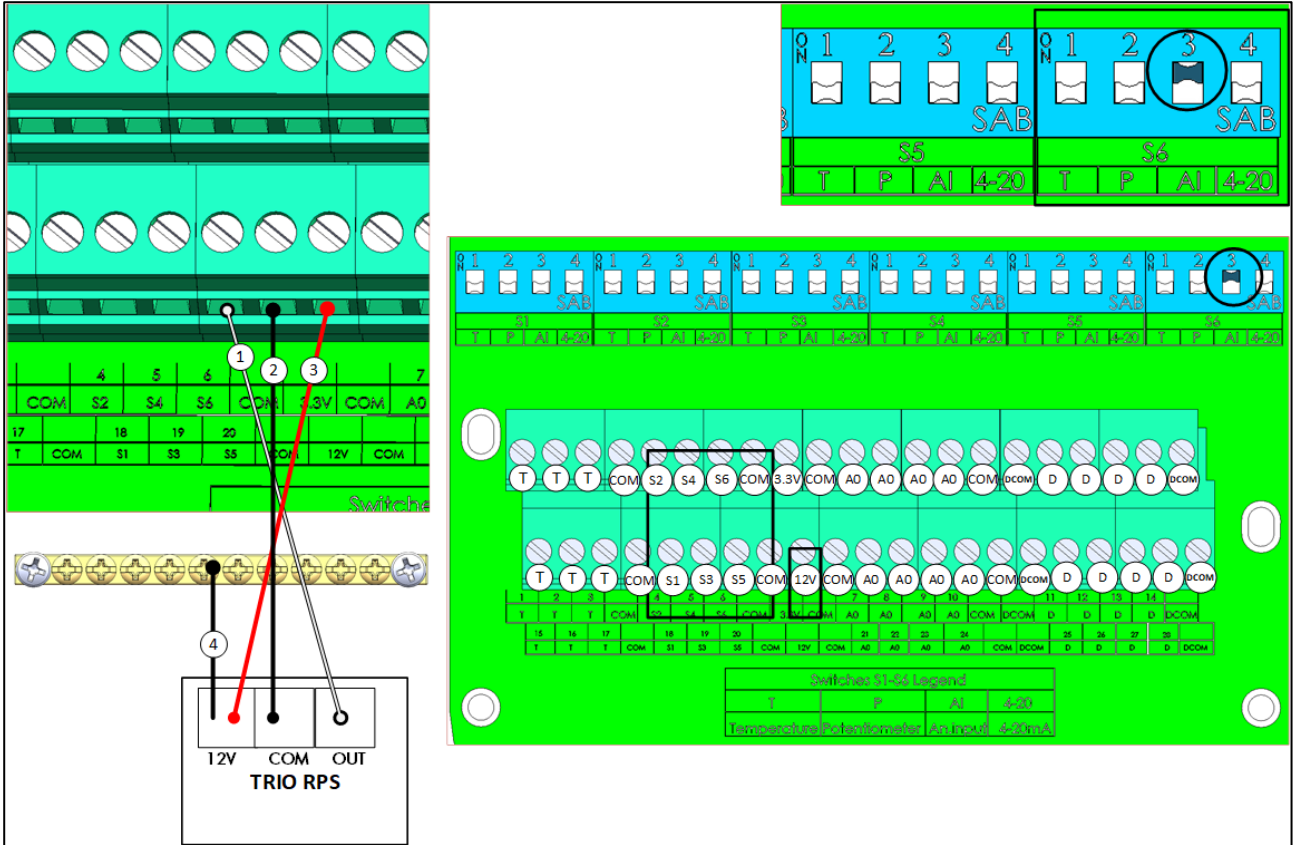
图 27: RPS接线
