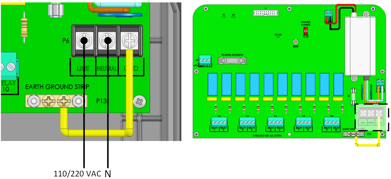
图 38: 电源端口
