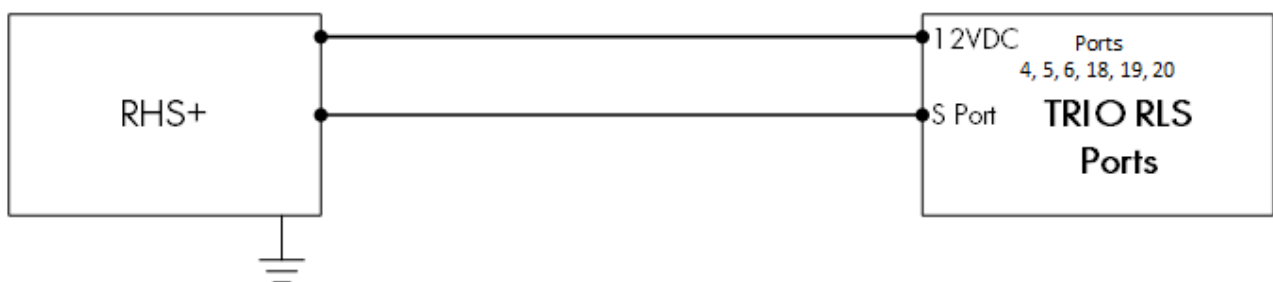
图 26: 接线图 RLS
