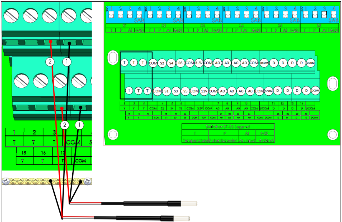
图 16: RTS 线
