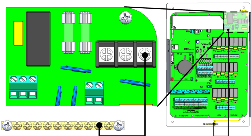
图 50: 接地
