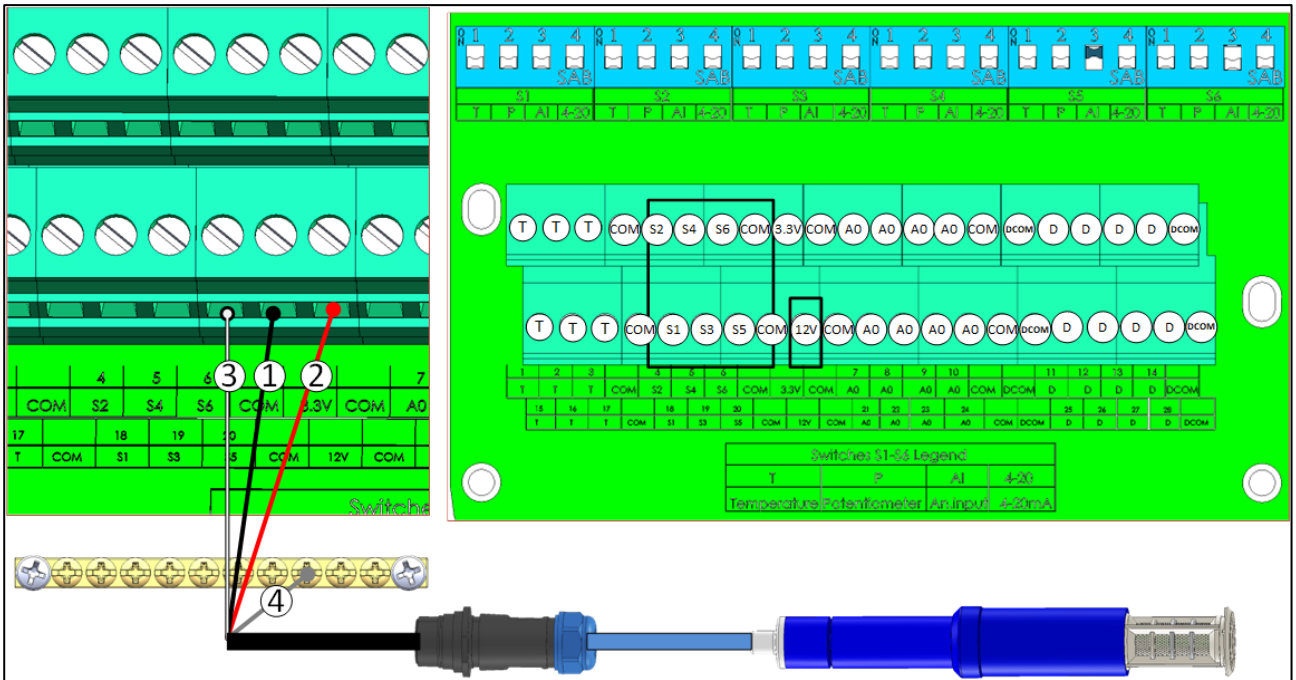
图19: RHS+ 布线
