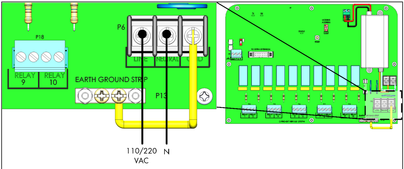
图 55: 电源端口
