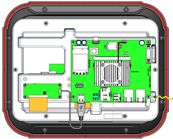
图 42: Trio CPU 面板 (后视图)
