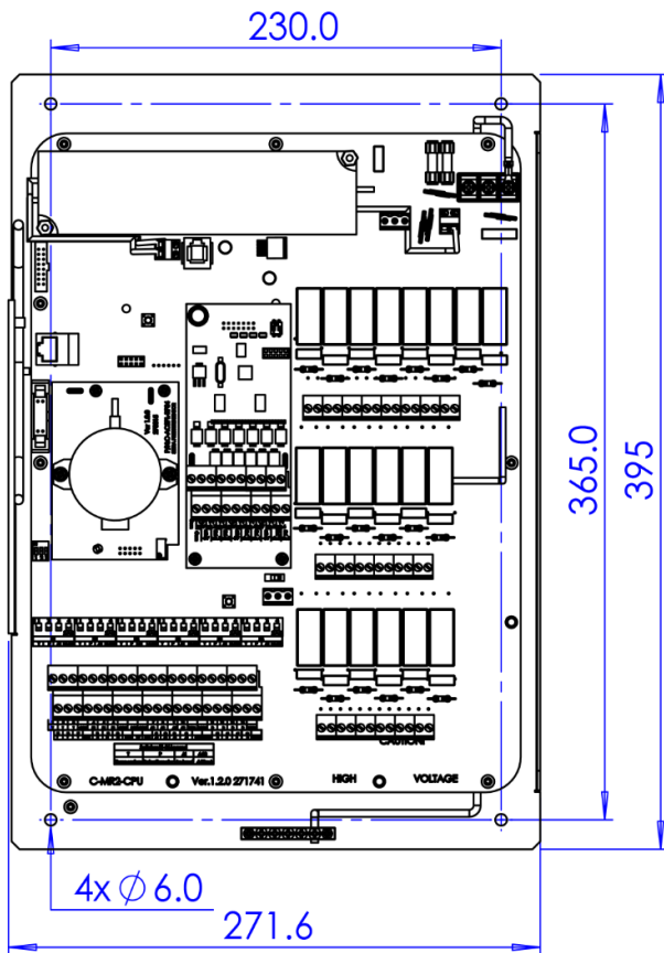
图 45: 后面板尺寸
