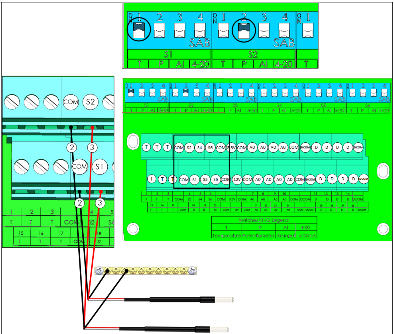
图 18: RTS S Port 线
