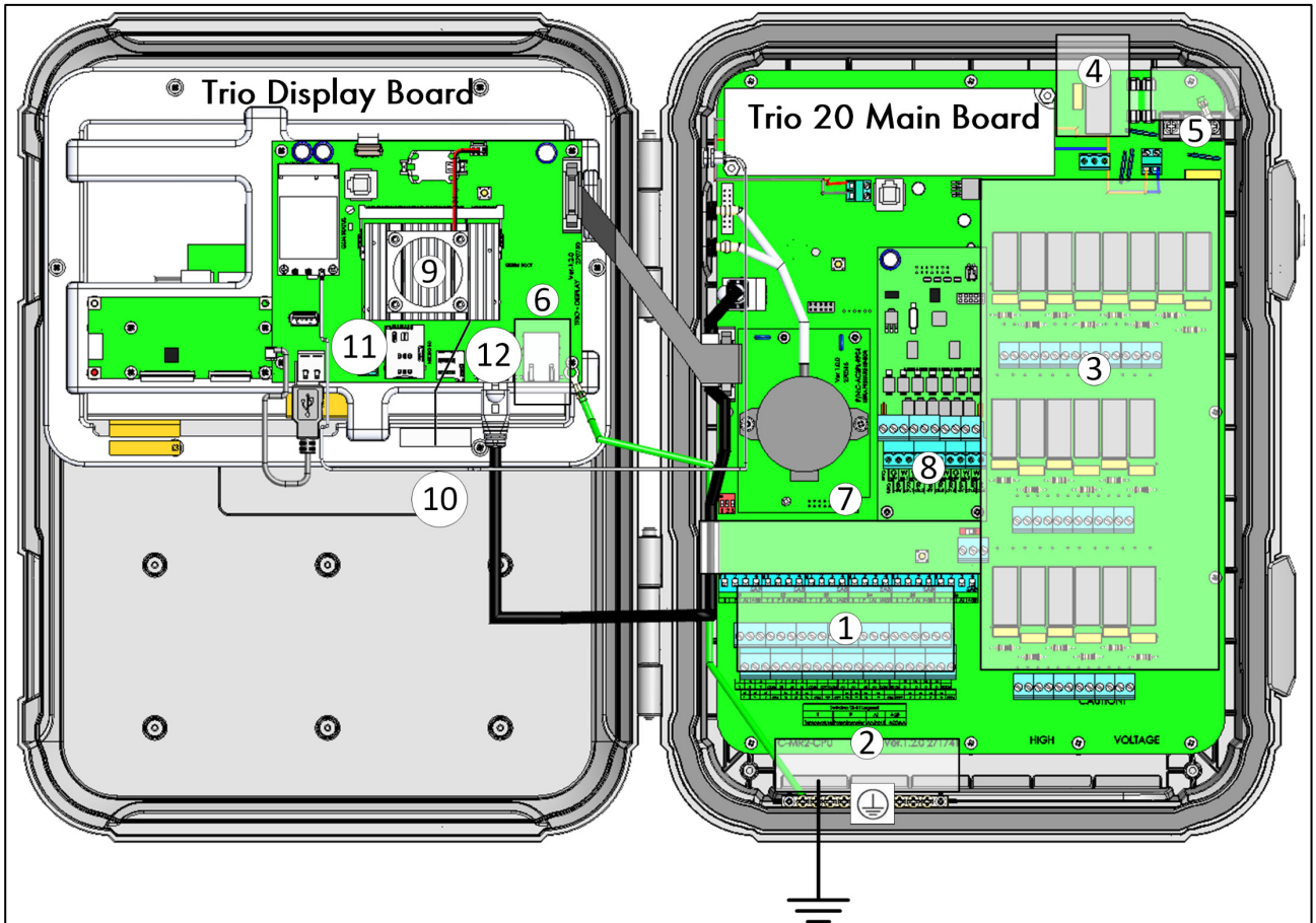
图2: 电路板布局 (转换文本)
