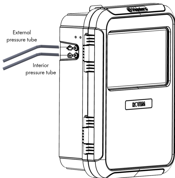
图 32: 静态压力软管 (转换文本)
