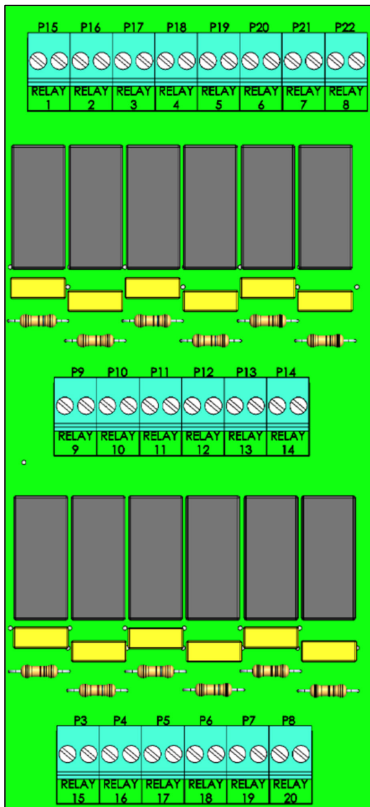
图6: 继电器和端口编号
