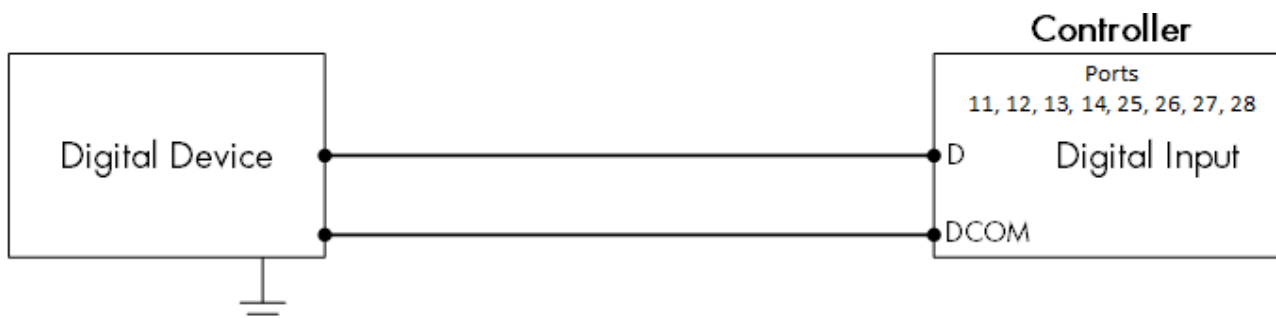
图 13: 数字设备接线图 (转换文本)
