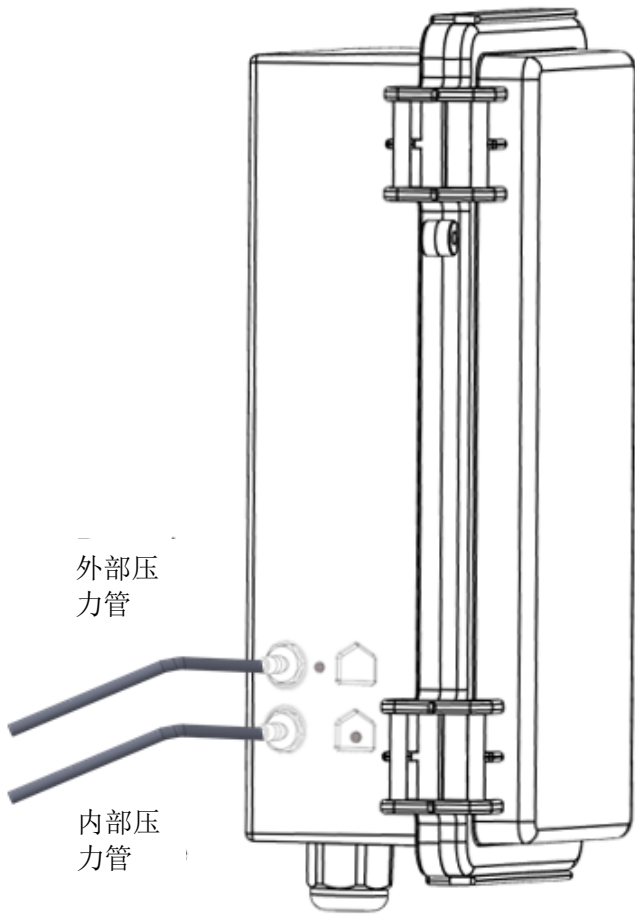
图 29: RPS压力管
