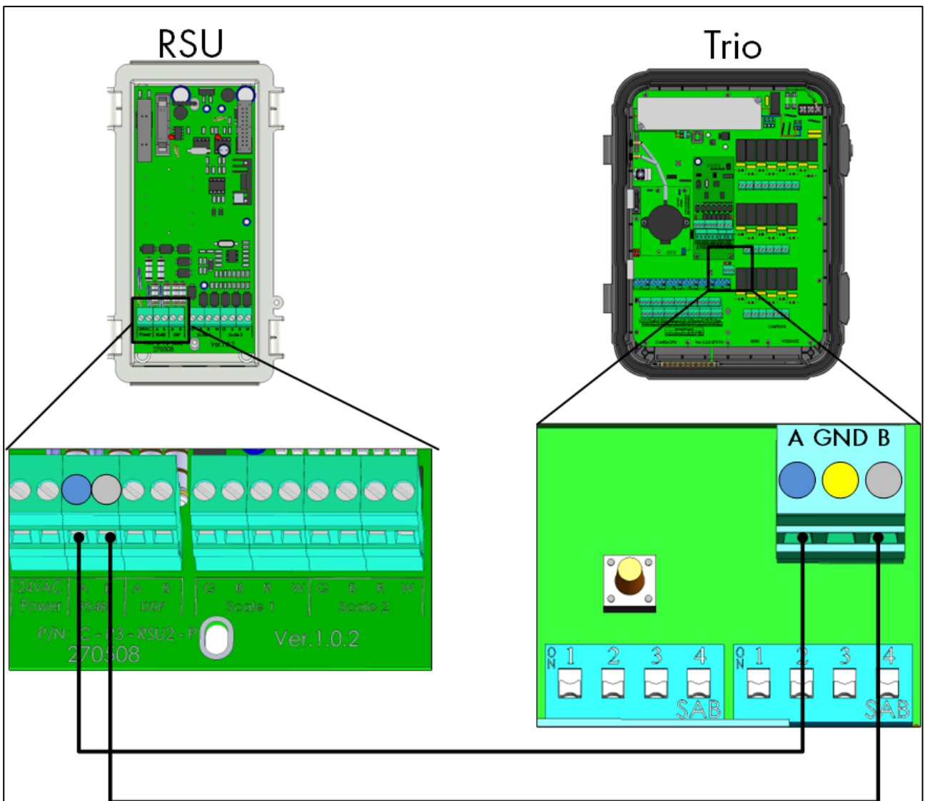
图 31: Trio 和 RSU 的接线图。
