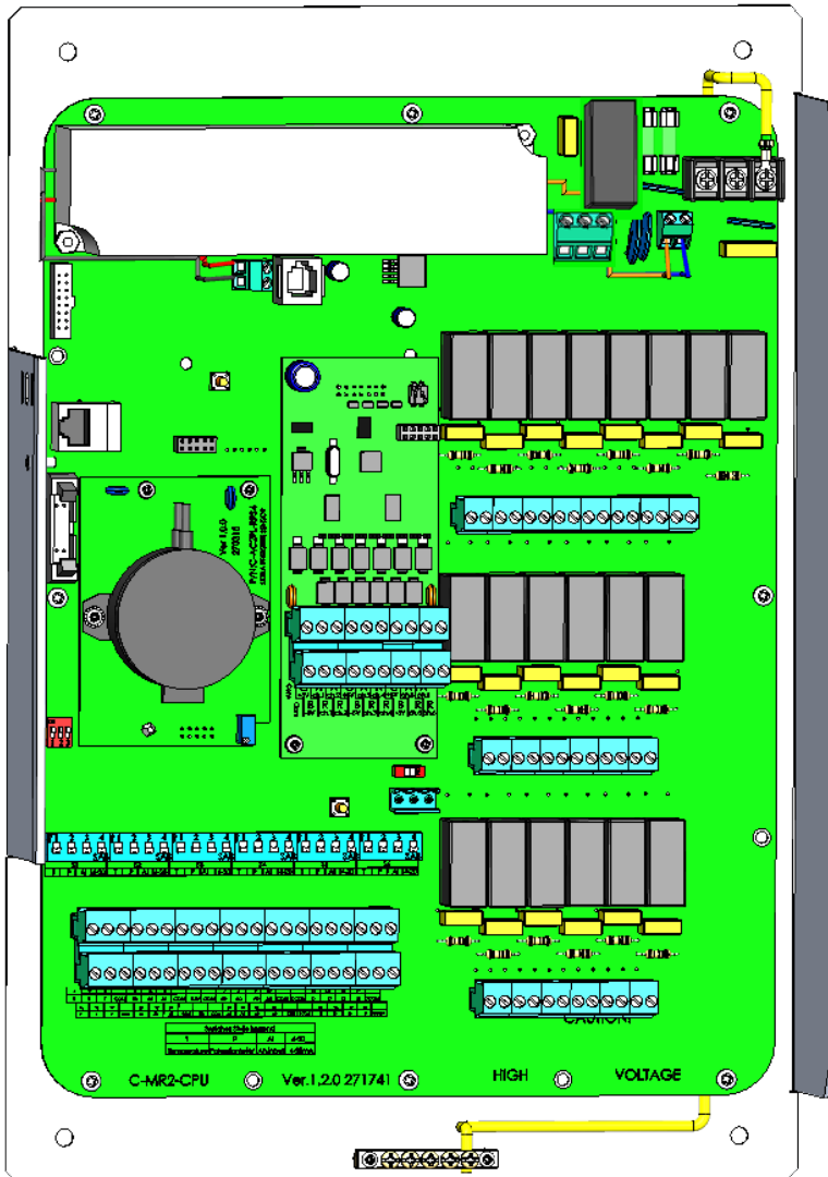
图 43: Trio 继电器面板 (正视图)
