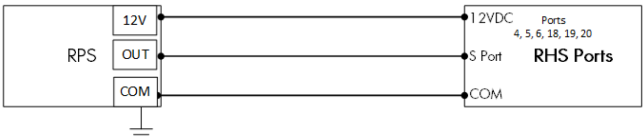
图 28: RPS 接线示意图
