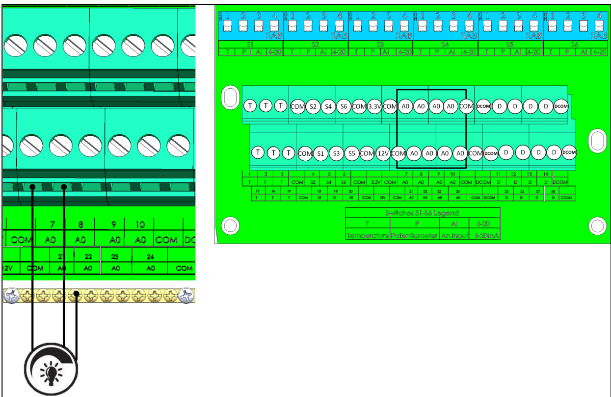
图10: 调光设备
