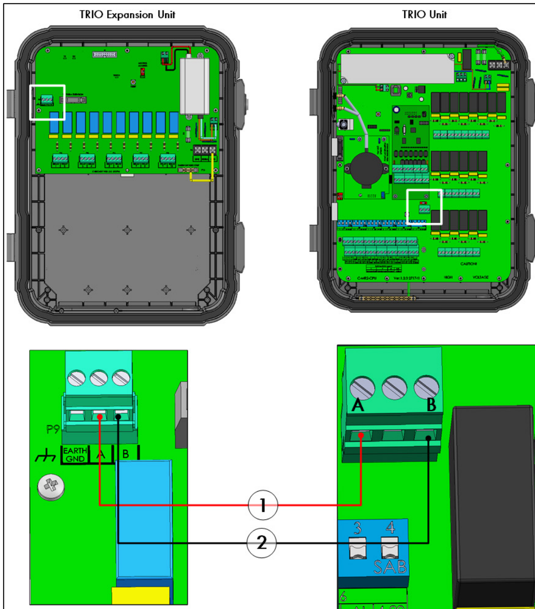
图 35: 接线图
