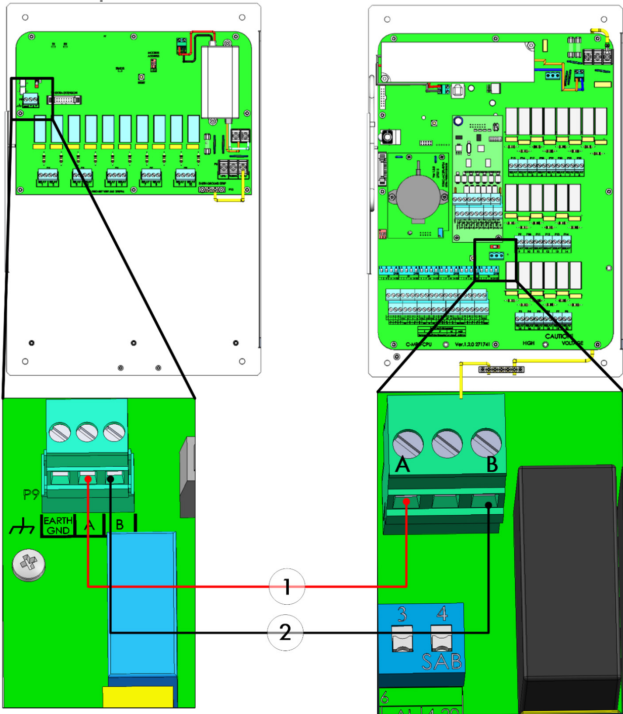
图 54: 面板安装/扩展面板安装接线
