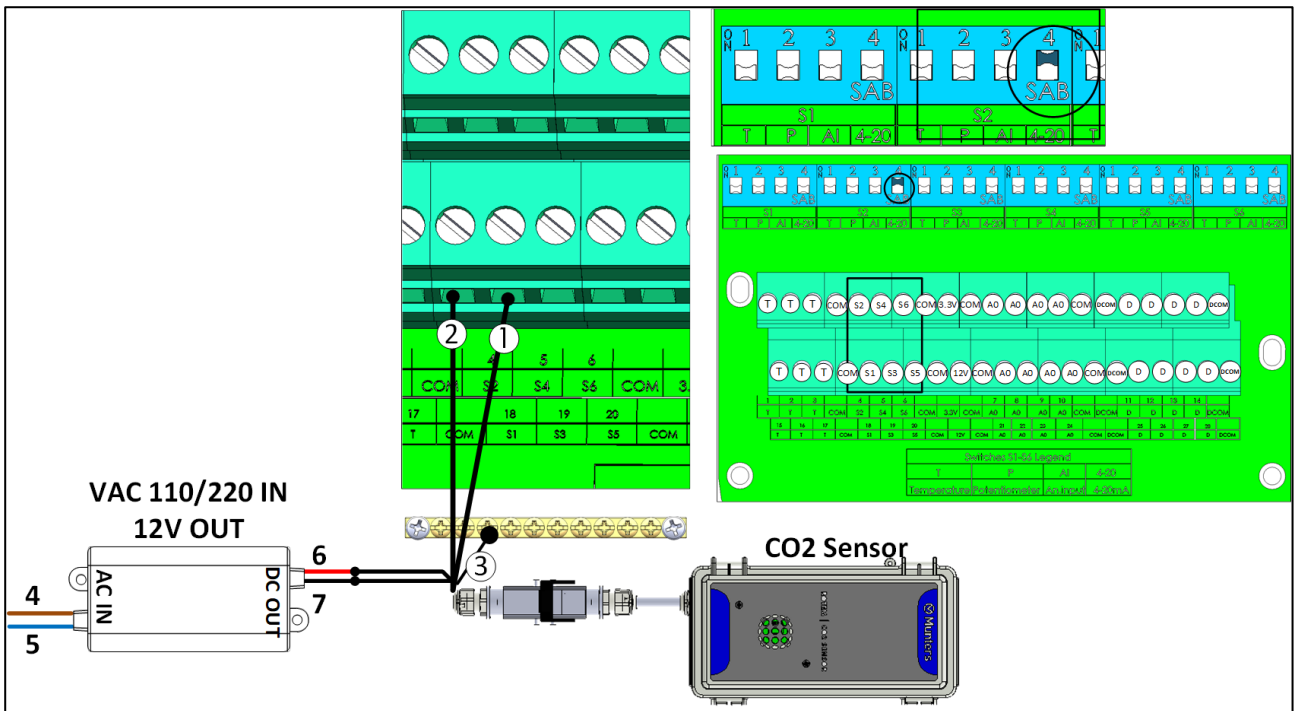
图 14:二氧化碳传感器布线（转换颜色）
