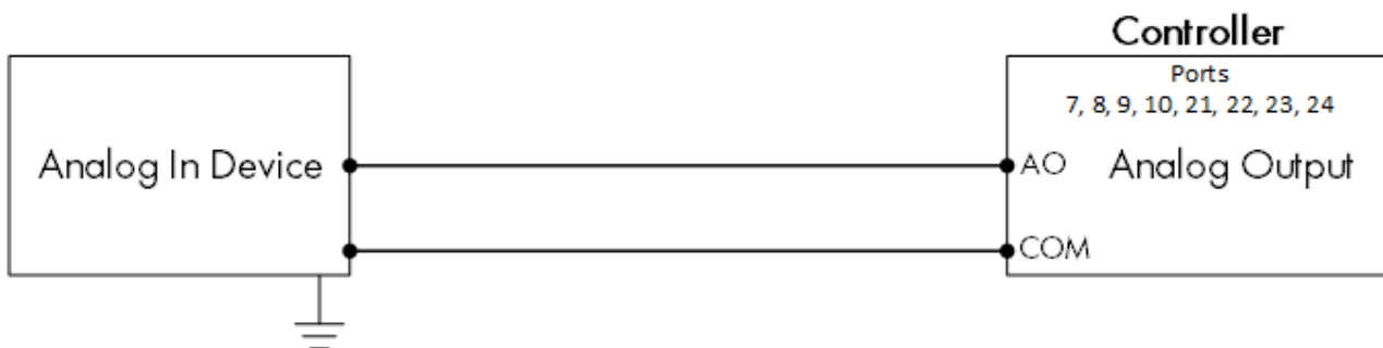
图 11: 模拟设备接线图 (转换文本)
