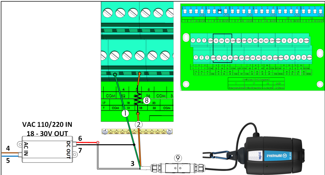
图 23: 氨气传感器接线
