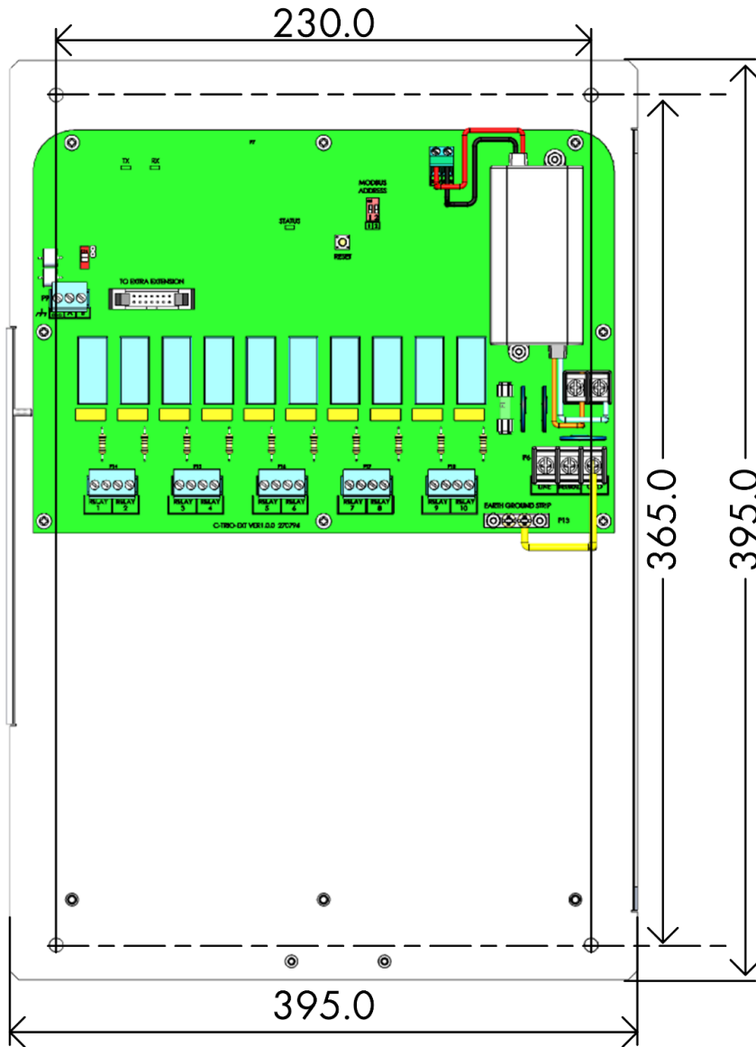
图 52: 扩展后面板尺寸
