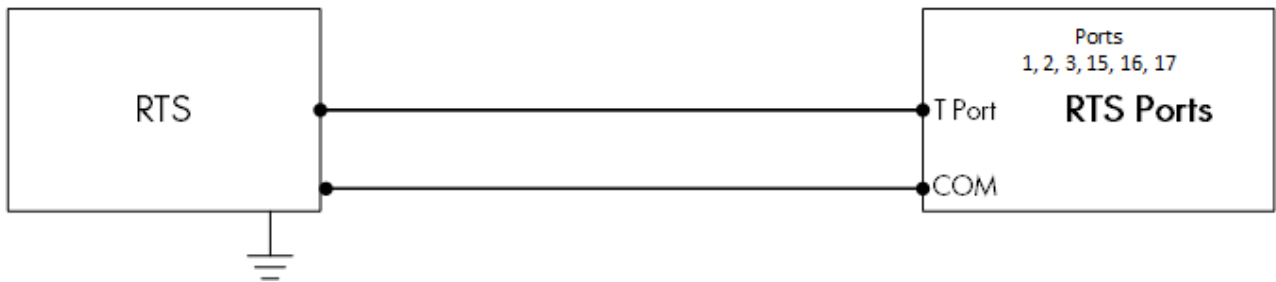
图 17: RTS 接线图
