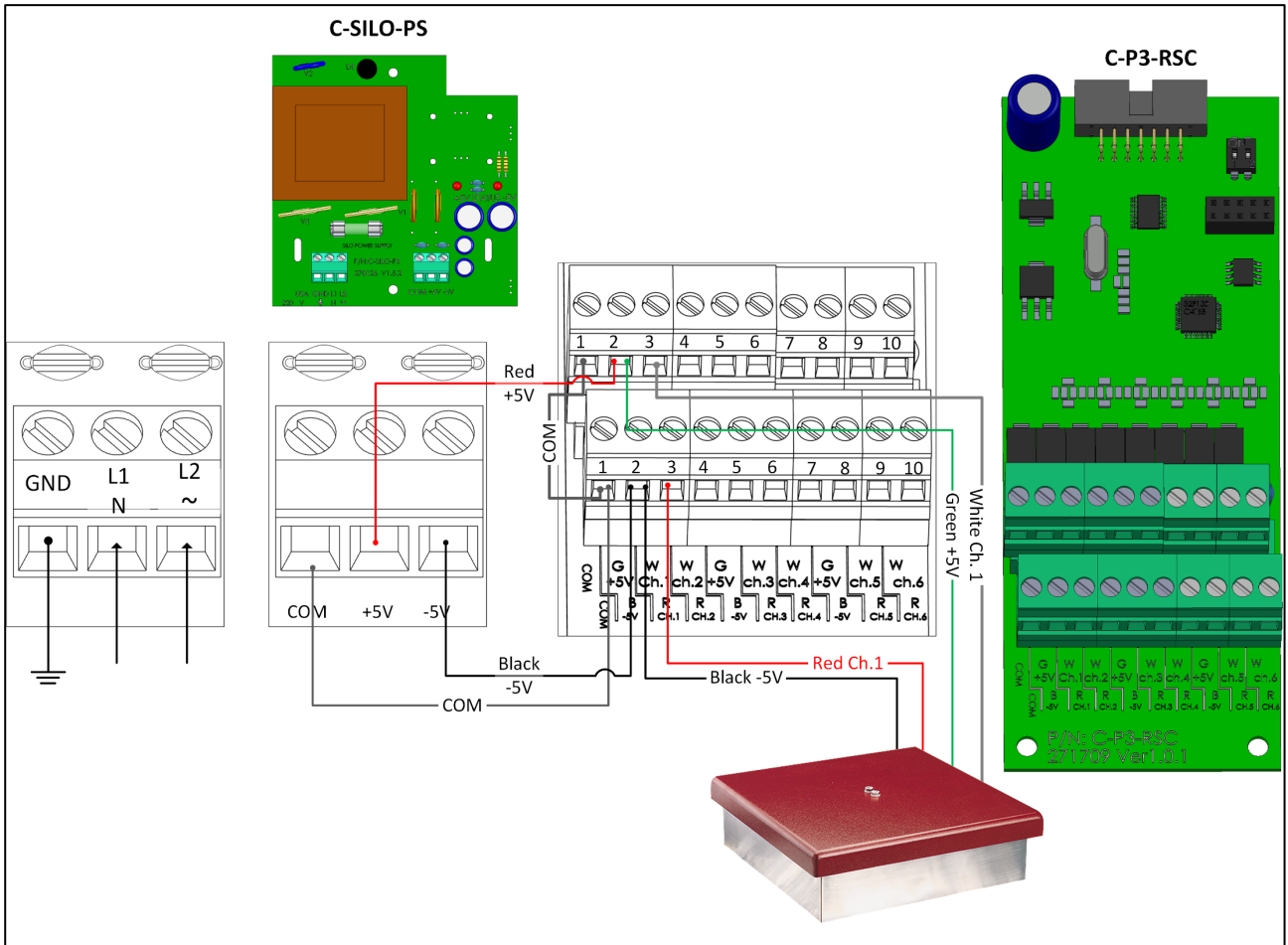
图 30: 称重卡接线到电源和鸡秤
