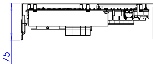
图 46: 后面板深度尺寸
