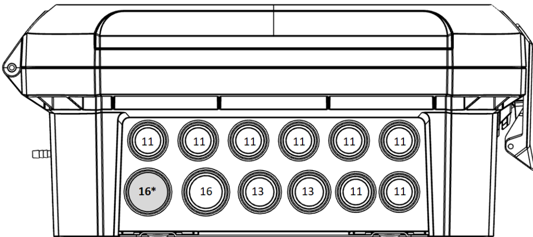
图 1：鸡管家TRIO 预留挡片和PG 螺纹尺寸
