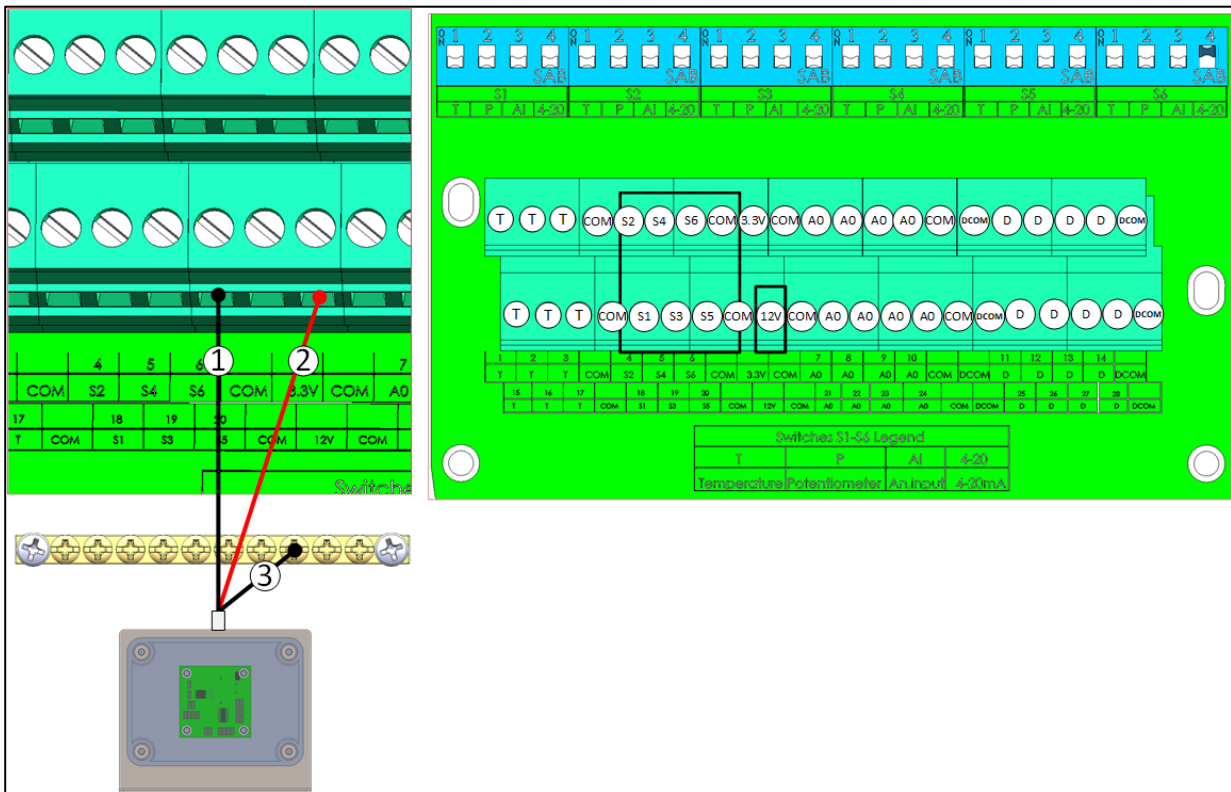
图 25: 光照传感器接线
