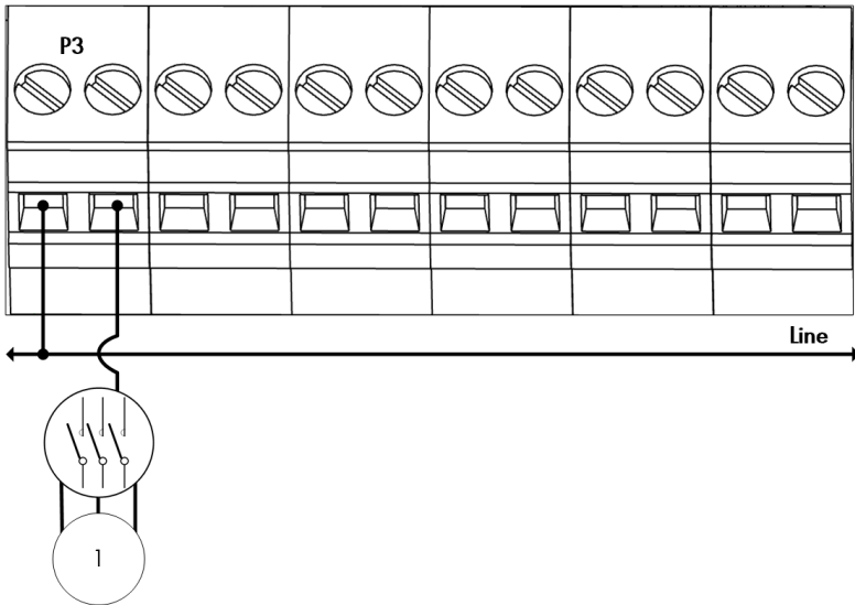
图5: 继电器接线细节图
