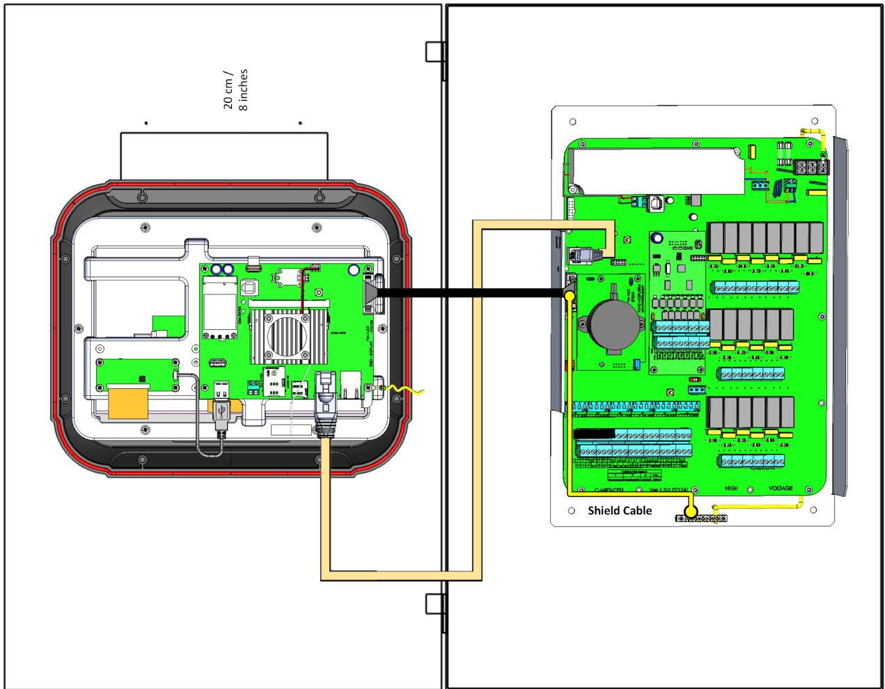
图 48: 面板安装，机柜打开（尺寸不按比例）
