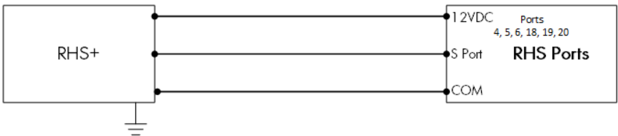
图20: RHS+ 传感器接线图 (转换文本)
