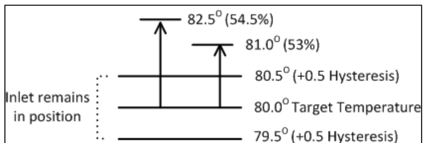
图26: 图解风门开启的滞后
