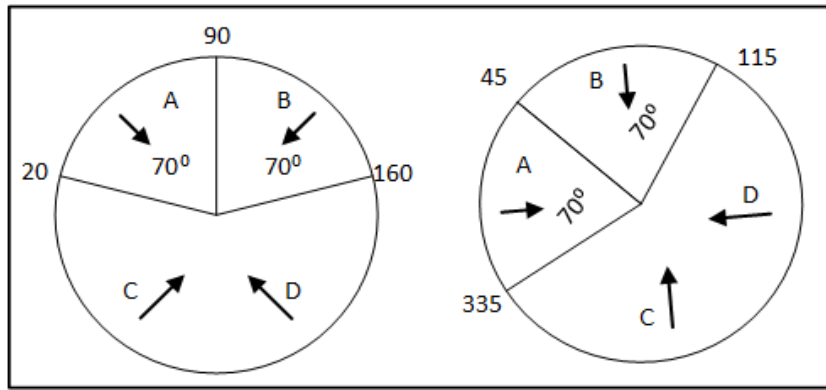
Figure 9: 风向传感器解说, 6.19 版本
