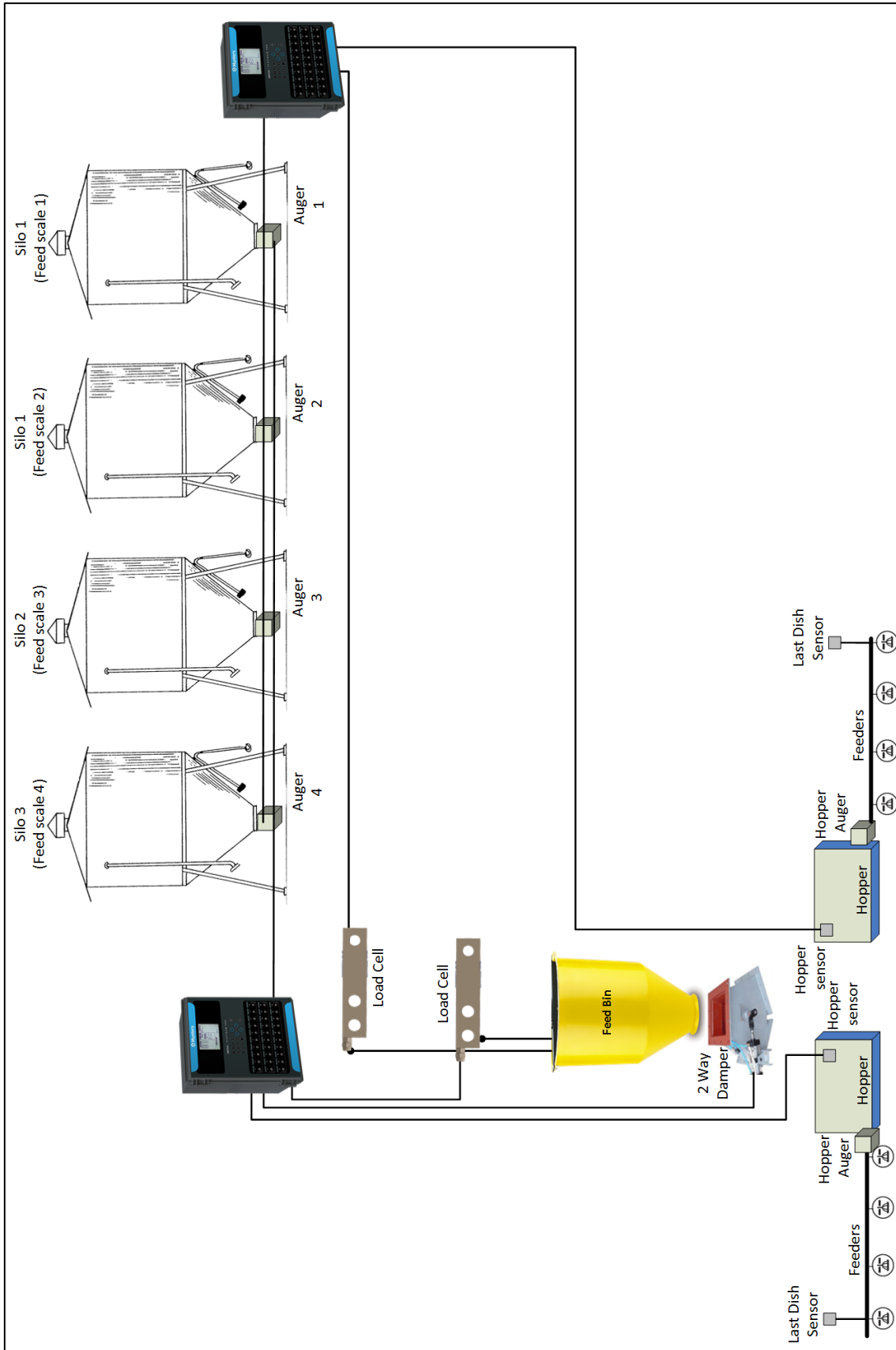
图10: 料称图示
