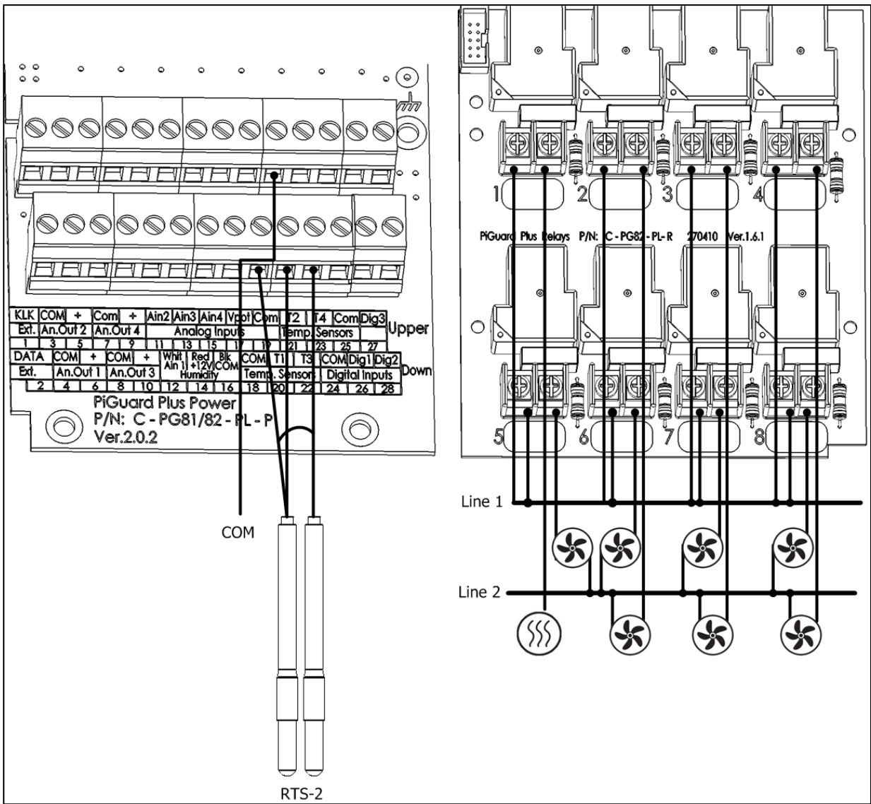
图 12: Pig Guard Plus 接线示意图(继电器,温度传感器)
