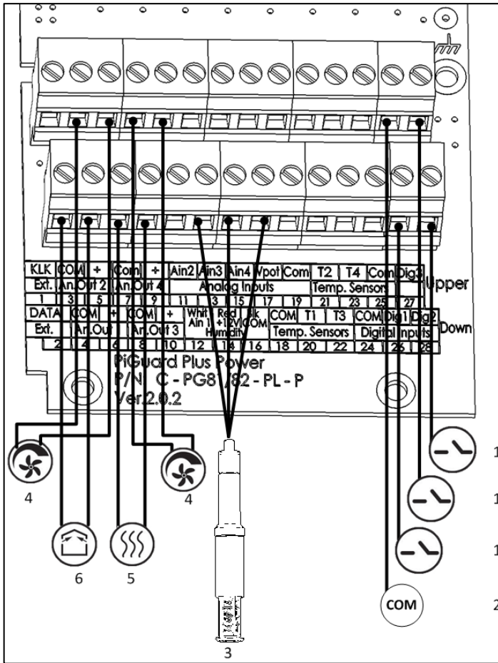
图 9: Pig Guard Plus接线示意图(模拟输出, 电源, 变速风机, 湿度传感器)
