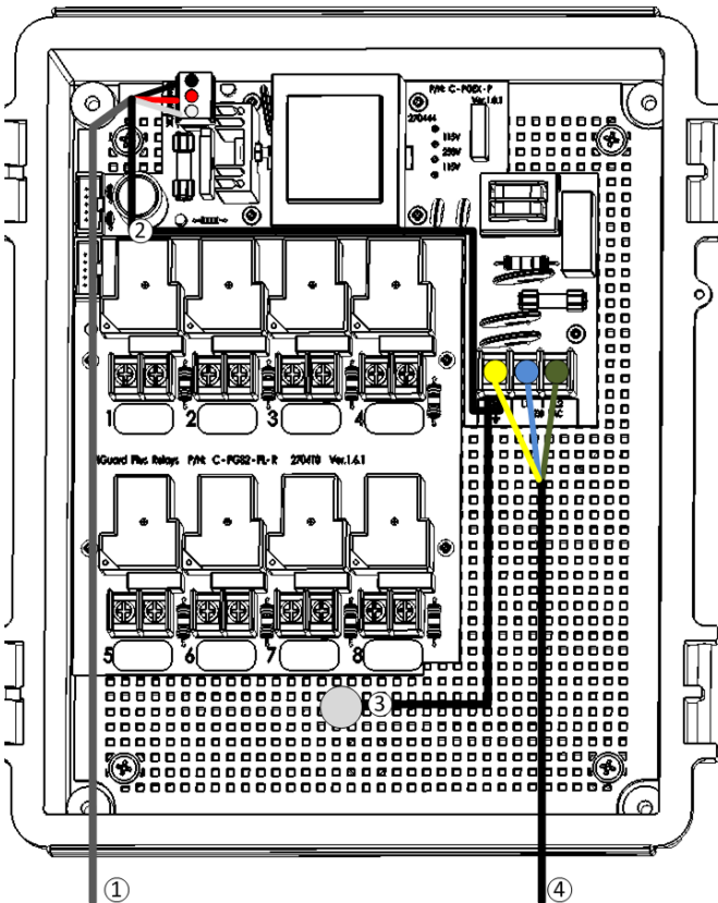
图 15: 扩展盒布线
