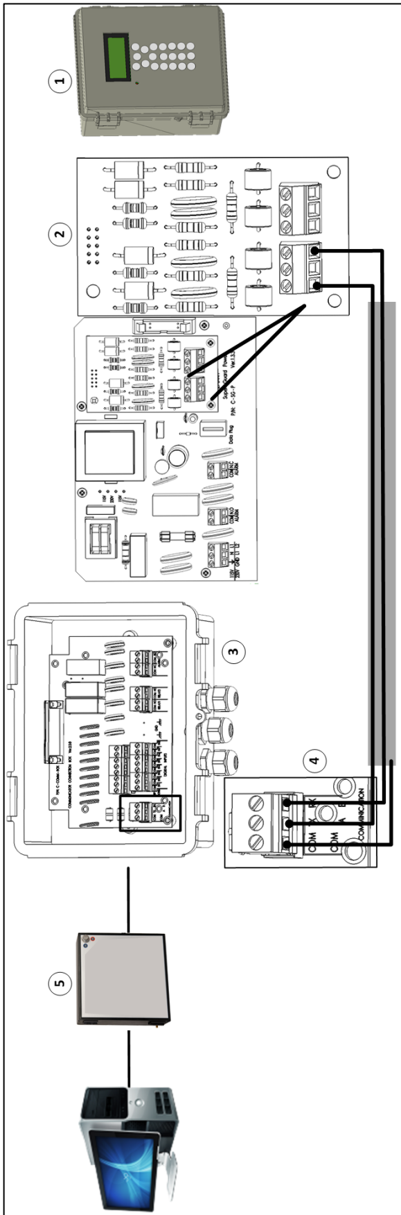
图 7: 通信接线示意图(Communicator)
