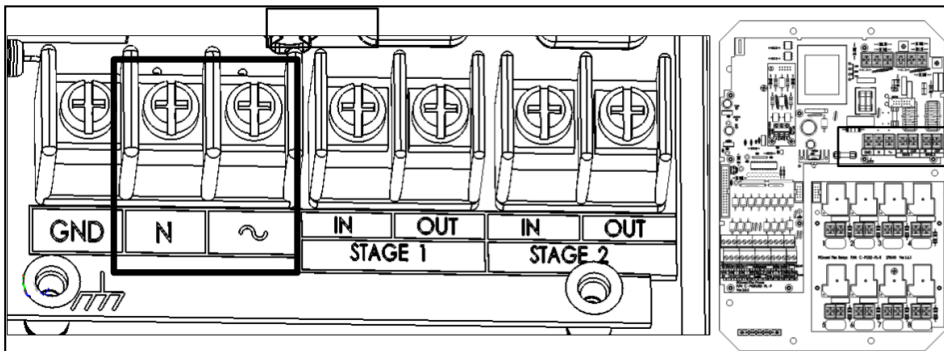
图 3: 电源输入端
